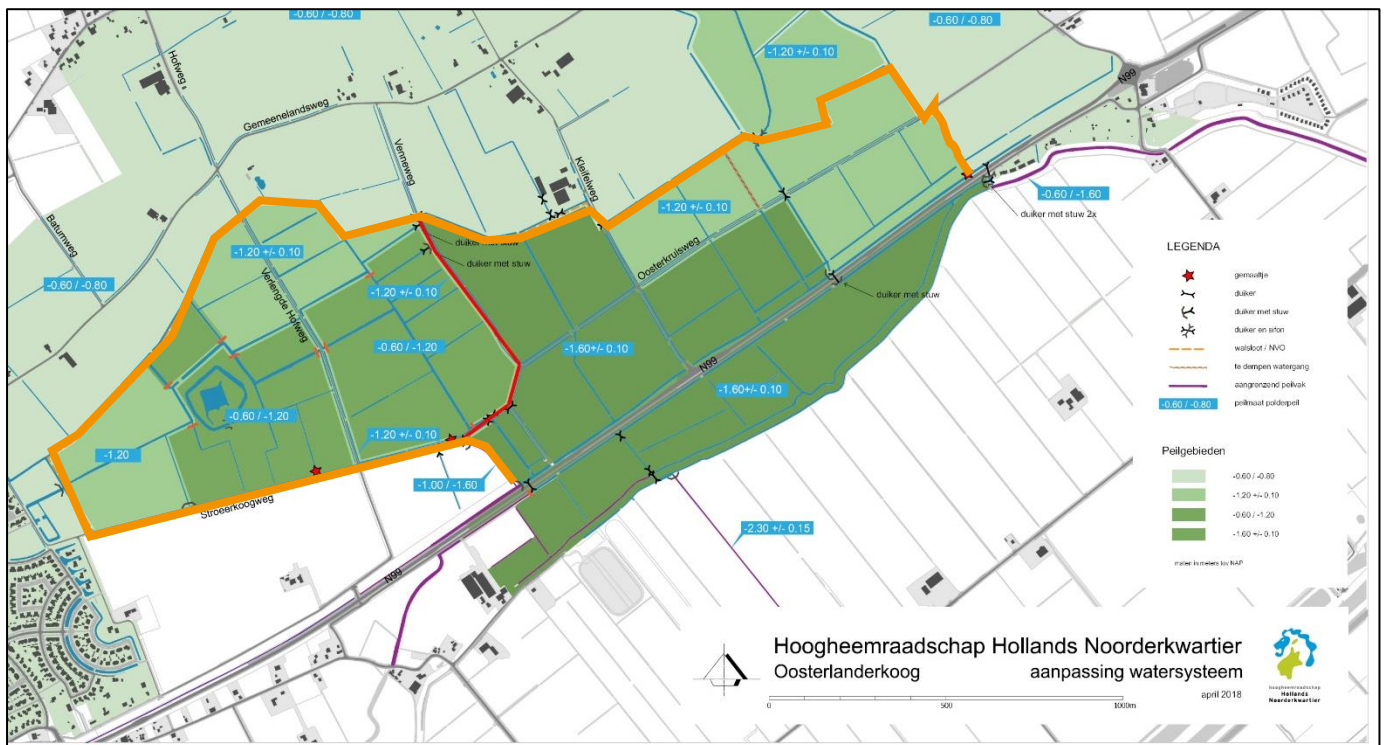
Figuur 2.3 Plangebied Oosterlanderkoog. Bij de rode en oranje lijn wordt de sloot verbreed.
