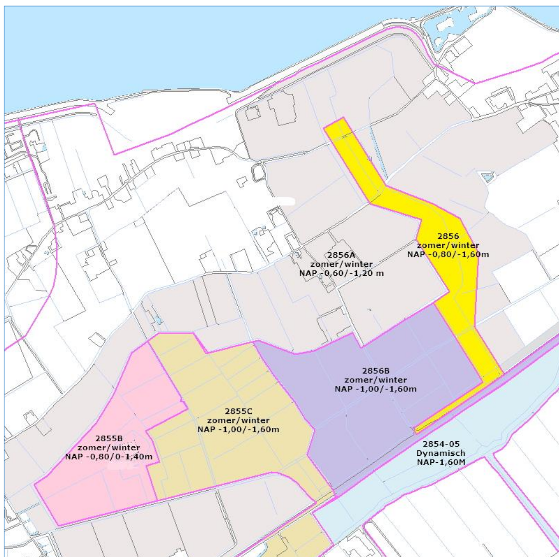
Figuur 63: Huidige peilenkaart
