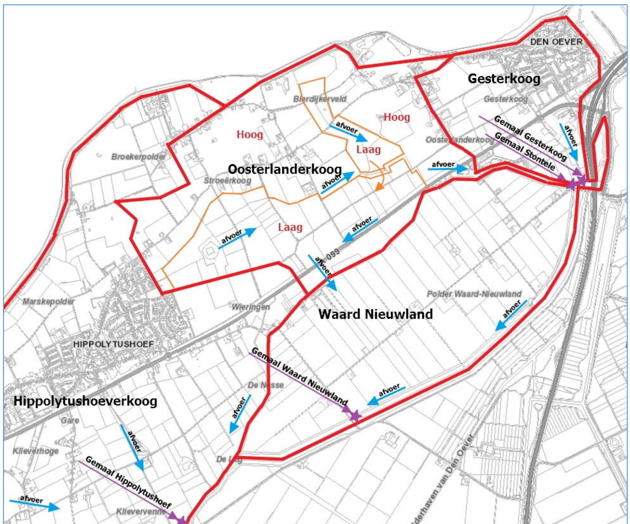
Figuur 7: Afvoerdeling naar de diverse gemalen
