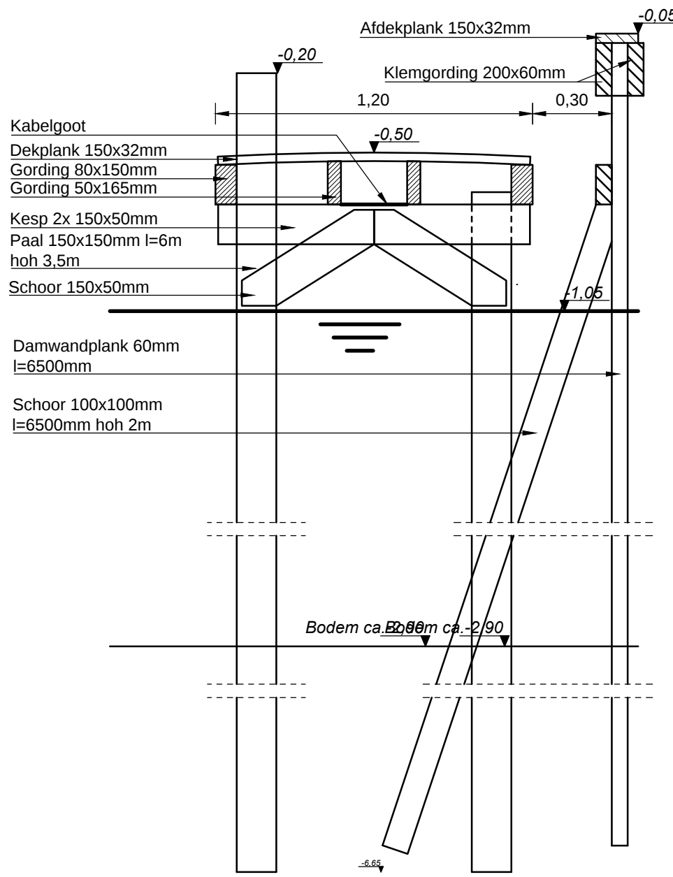
STEIGER 1,2M BREED SCHAAL: 1:20
