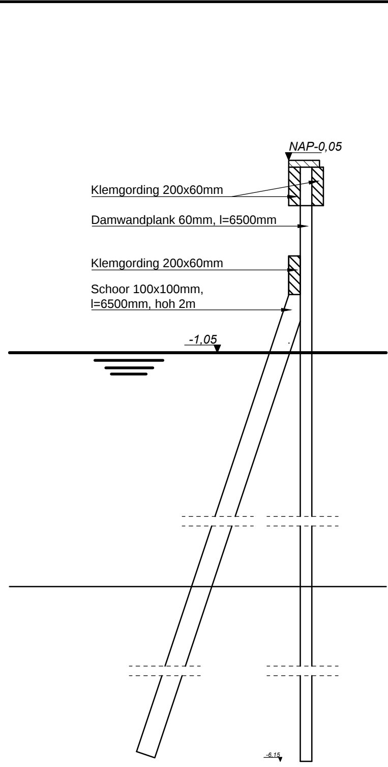
GOLFKERING SCHAAL: 1:20
