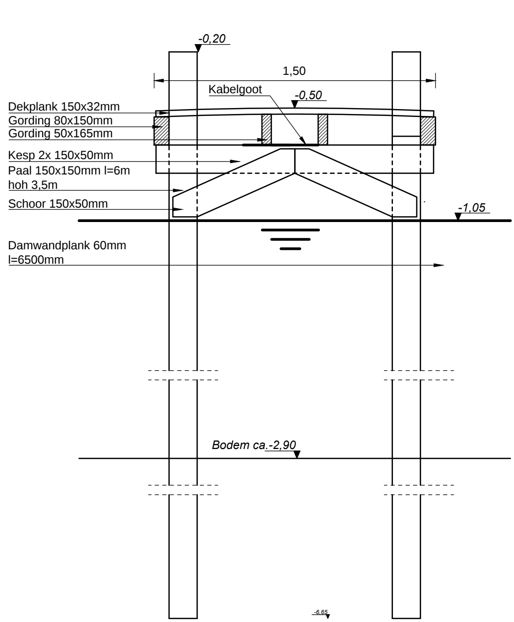
STEIGER 1,5M BREED ZONDER GOLFKERING SCHAAL: 1:20
