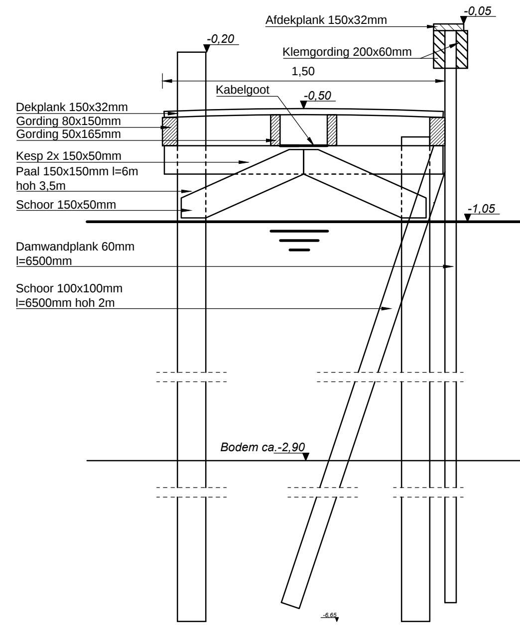
STEIGER 1,5M BREED SCHAAL: 1:20
