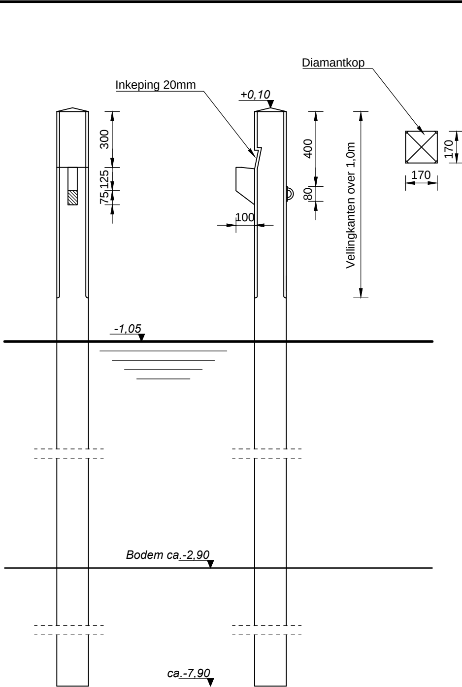
ACHTERPALEN VOOR-, ZIJ- EN BOVENAANZICHT SCHAAL: 1:20
