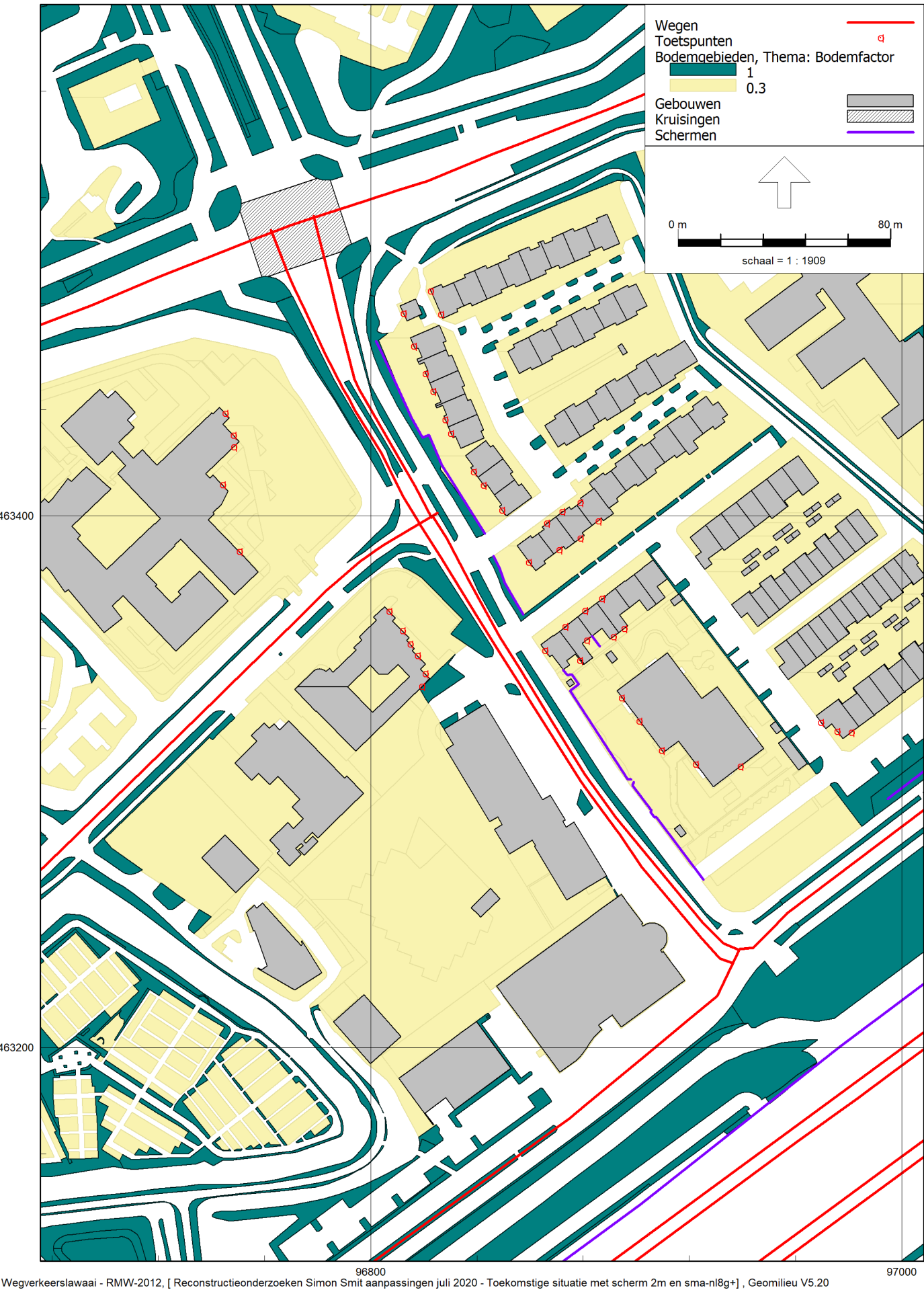
Wegverkeerslawaaï - RMW-2012, [ Reconstructieonderzoeken Simon Smit aanpassingen juli 2020 - Toekomstige situatie met scherm 2m en sma-nl8g+ ] , Geomilieu V5.20
