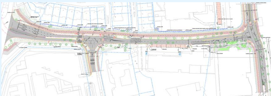
figuur 1: nieuwe inrichting Simon Smitweg
