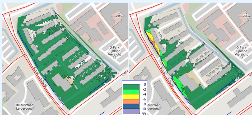
figuur 5: effect 2 meter hoog scherm op geluidsbelasting van Simon Smitweg (links: 1 e verdieping; rechts: begane grond)
