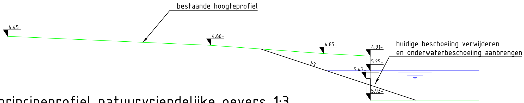
principeprofiel natuurvriendelijke oevers 1:3 SCHAAL 1 : 50
