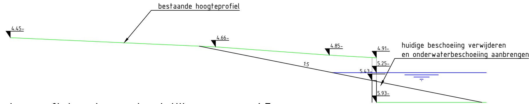
principeprofiel natuurvriendelijke oevers 1:5 SCHAAL 1 : 50
