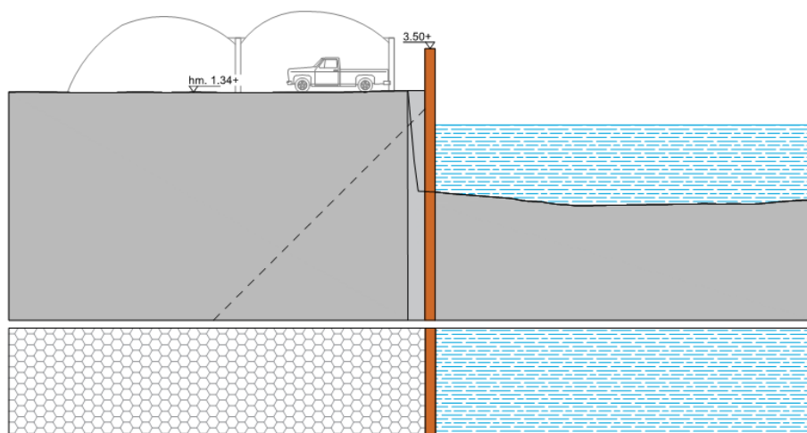
Figuur 2.19 Variant 4B: Dwarsprofiel met verhoogde damwand aan de Katwolderhaven (DP G)
