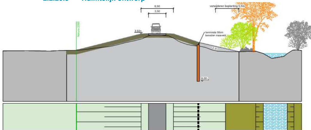
Figuur 2.47 Dwarsprofiel met groene kering en stabiliteitsscherm aan de binnenzijde. Beheerroute loopt onderlangs. Omwille van de dijkmaatregel, beheer en realisatie dient een deel van de binnendijkse NNN-bossingel gekapt te worden.
