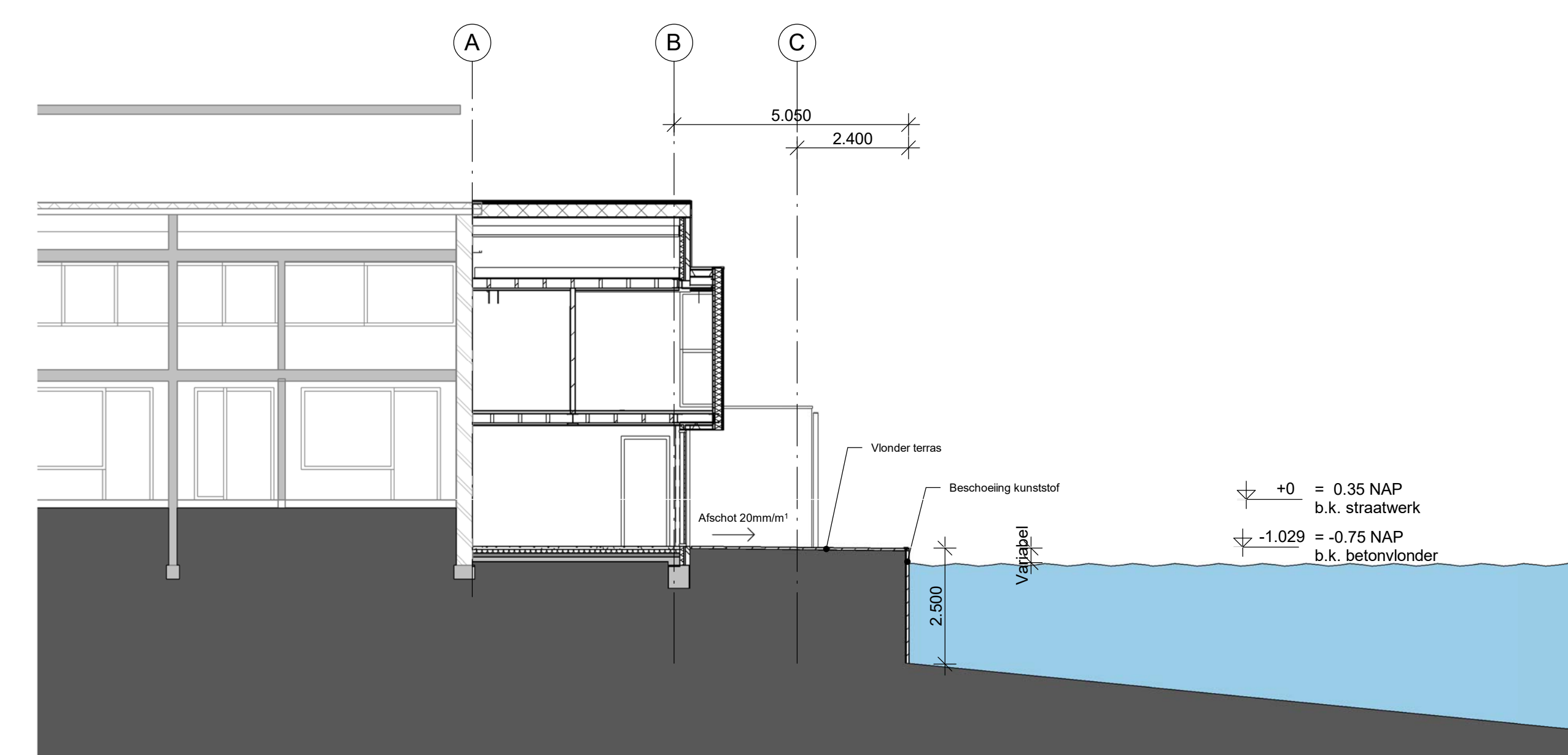
Doorsnede A beschoeiing Schaal: 1 : 100
