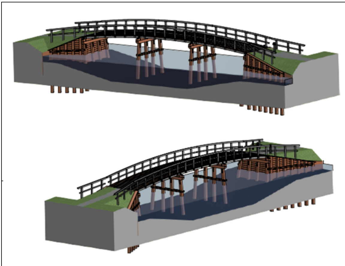
Figuur 2: ontwerp nieuwe brug
