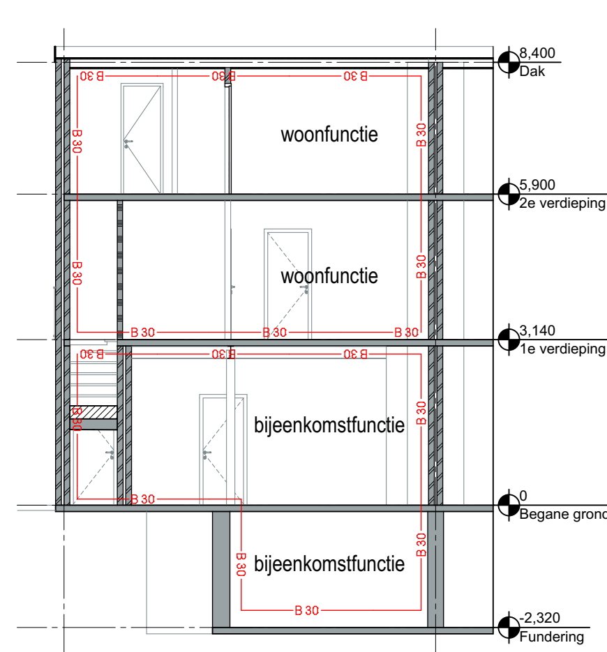
Doorsnede A-A
