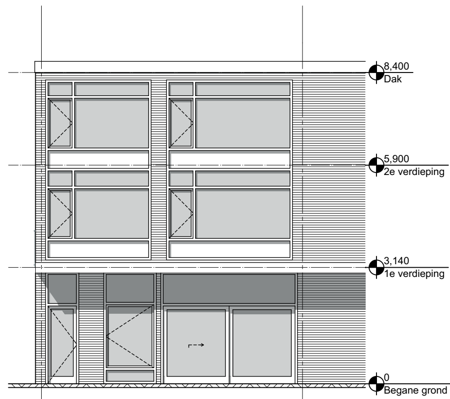
Voorgevel
