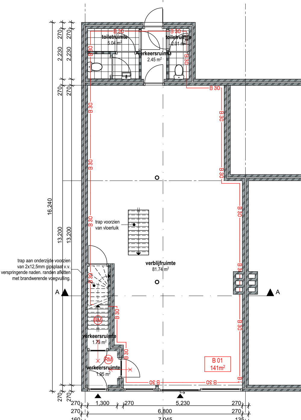
Begane grond
