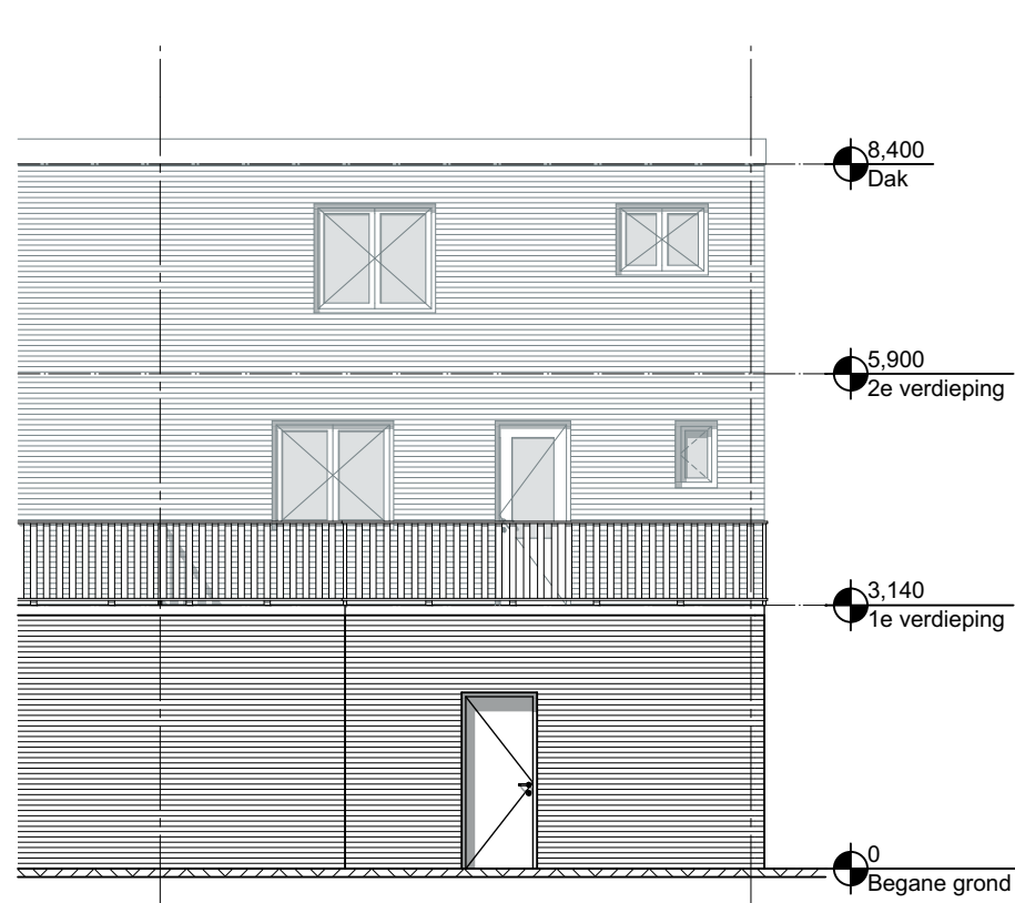
Achtergevel
