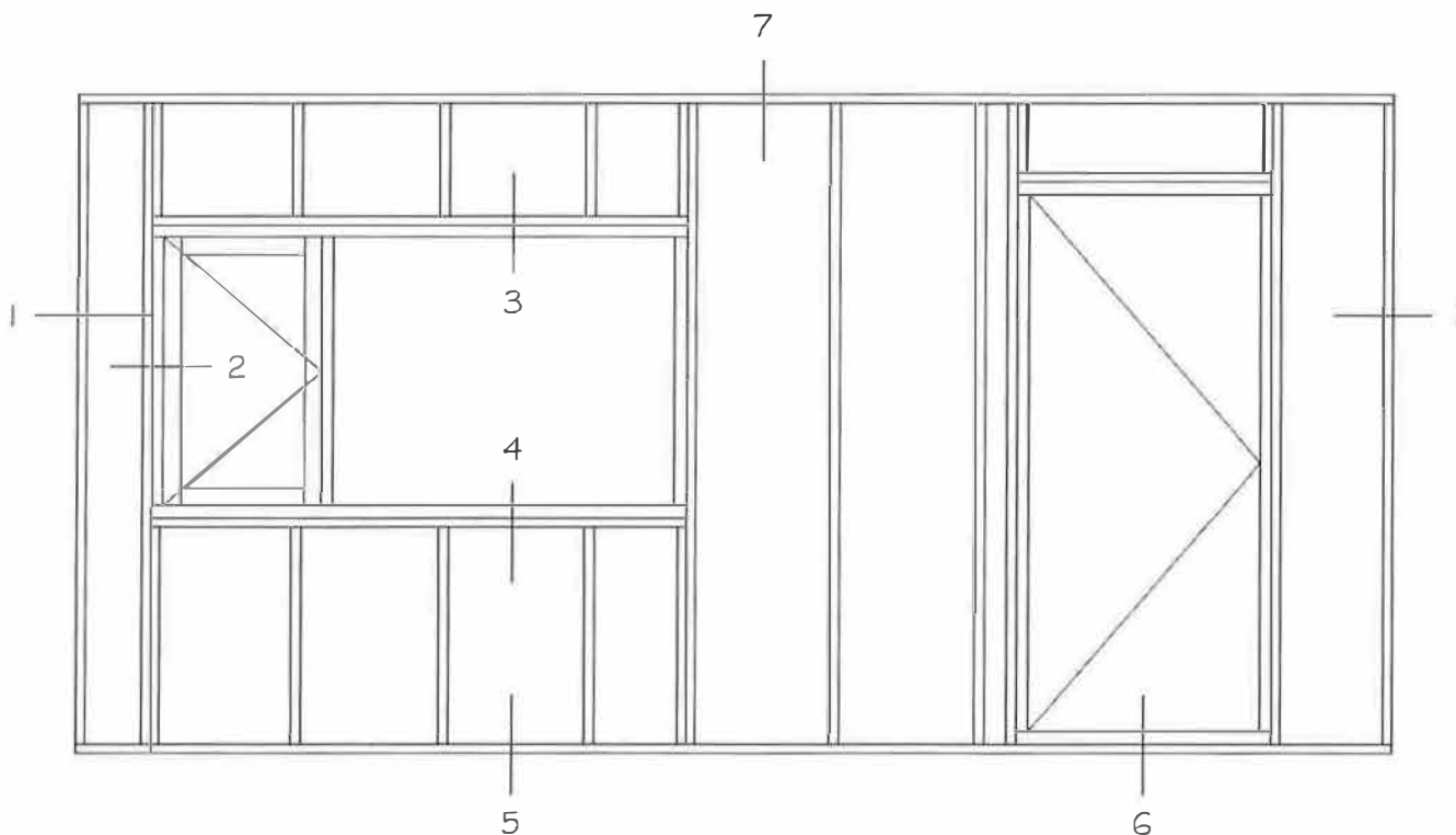
Bijlage 3 details gevelvullende elementen
