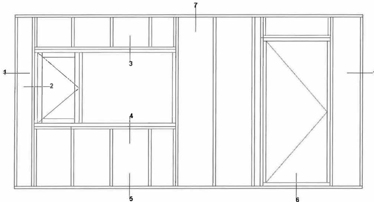
Bijlage 2A details binnenspouwblade I ligger
