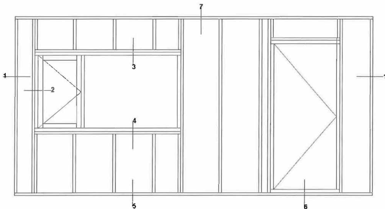
Bijlage 2 details binnenspouwbladen
