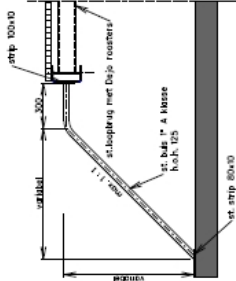
Zijaanzicht vuilrooster (alternatief bevestiging aan st. liggerbalk)
