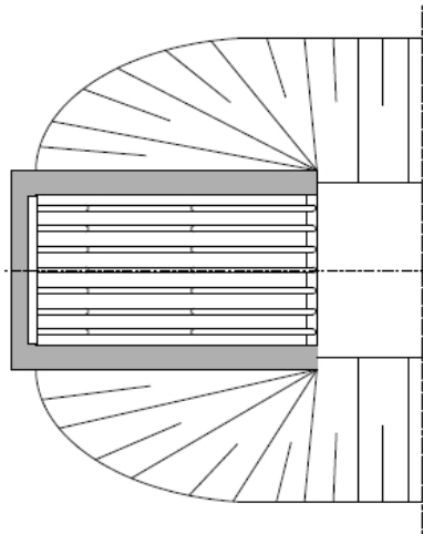
Bovenaanzicht vuilrooster
