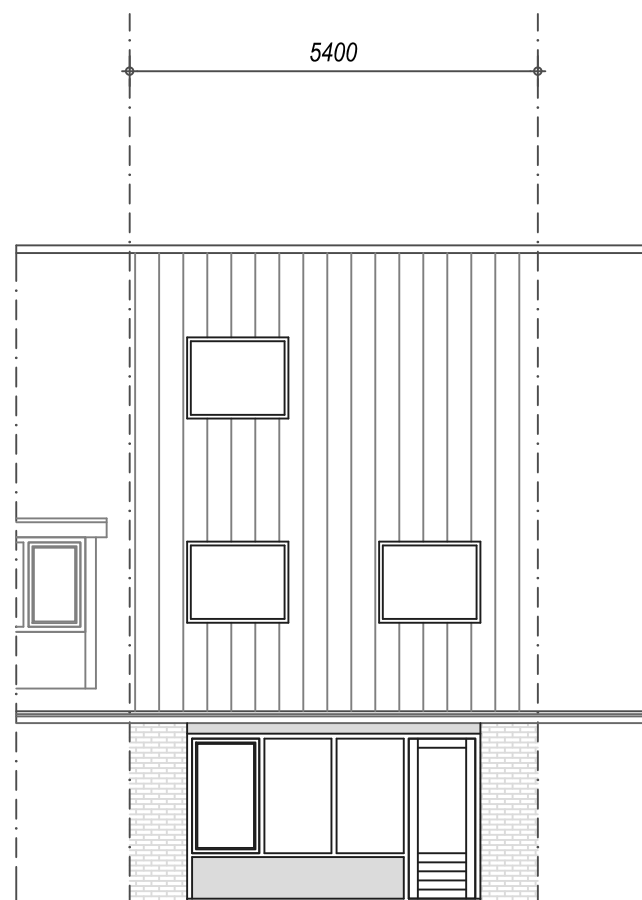
Achtergevel - bestaand
