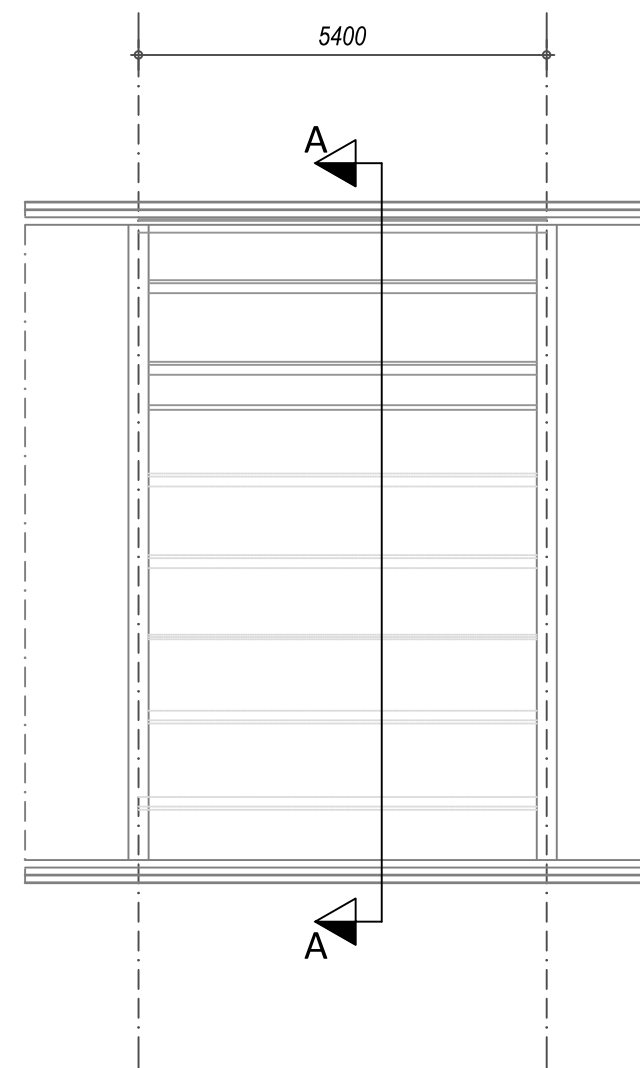
Kapplan - bestaand
