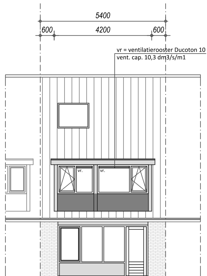
Achtergevel - nieuw
