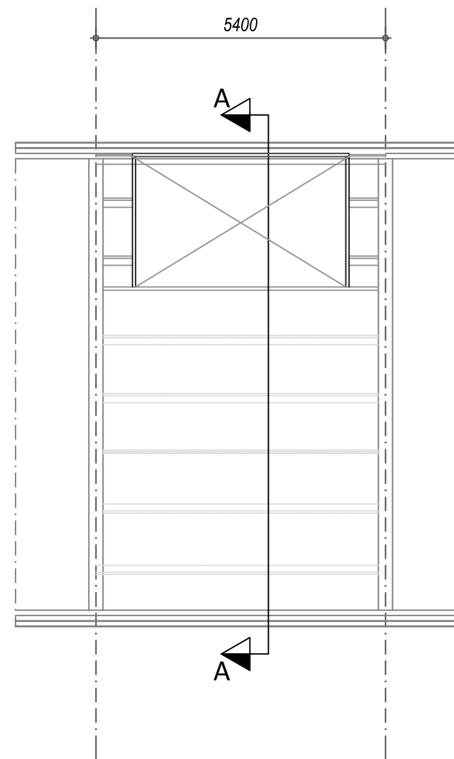
Kapplan - nieuw
