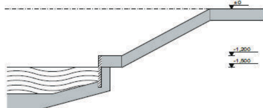
doorsnede A-A bestaand
