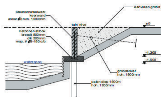
doorsnede A-A nieuw
