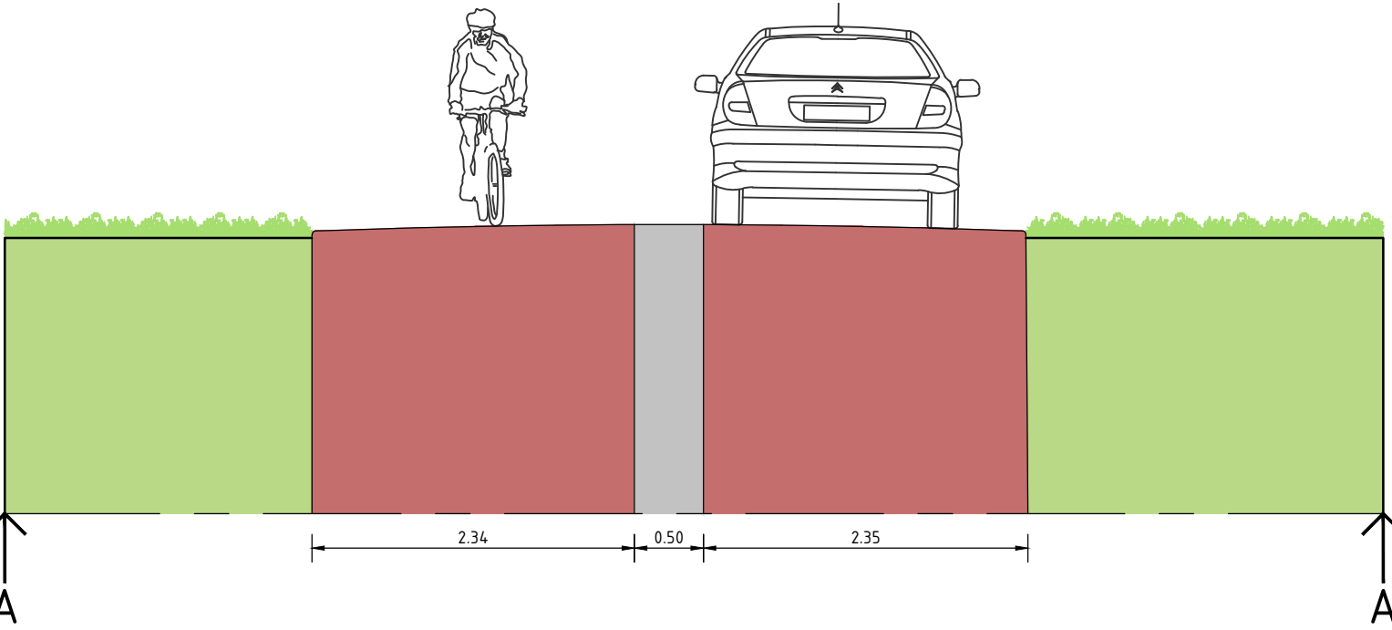
Dwarsprofiel: A-A Schaal: 1:50
