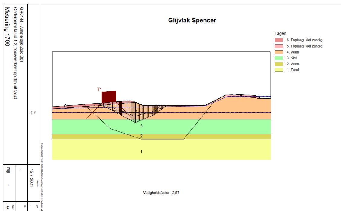
Figuur 4-3: Modellering stabiliteitsberekening sanering uitvoeringsfase – belasting op 3 m uit insteek talud (onderberm)
