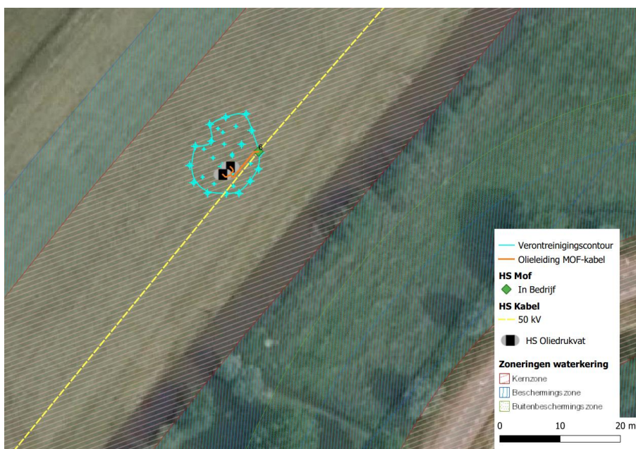
Figuur 1-2: Leggerprofiel (zonnering) Amsteldijk-Zuid nabij nr. 201
