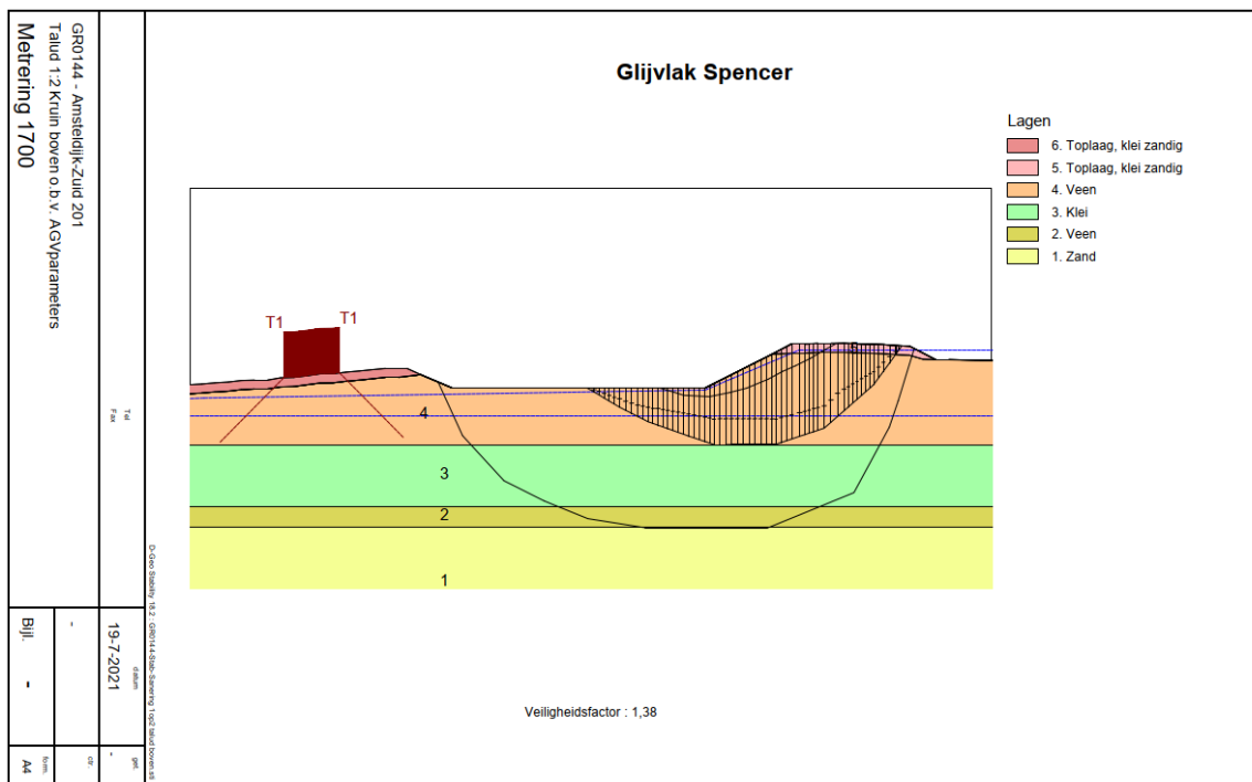
Figuur 4-2: Modellering stabiliteitsberekening sanering uitvoeringsfase – talud 1:2 kruin
