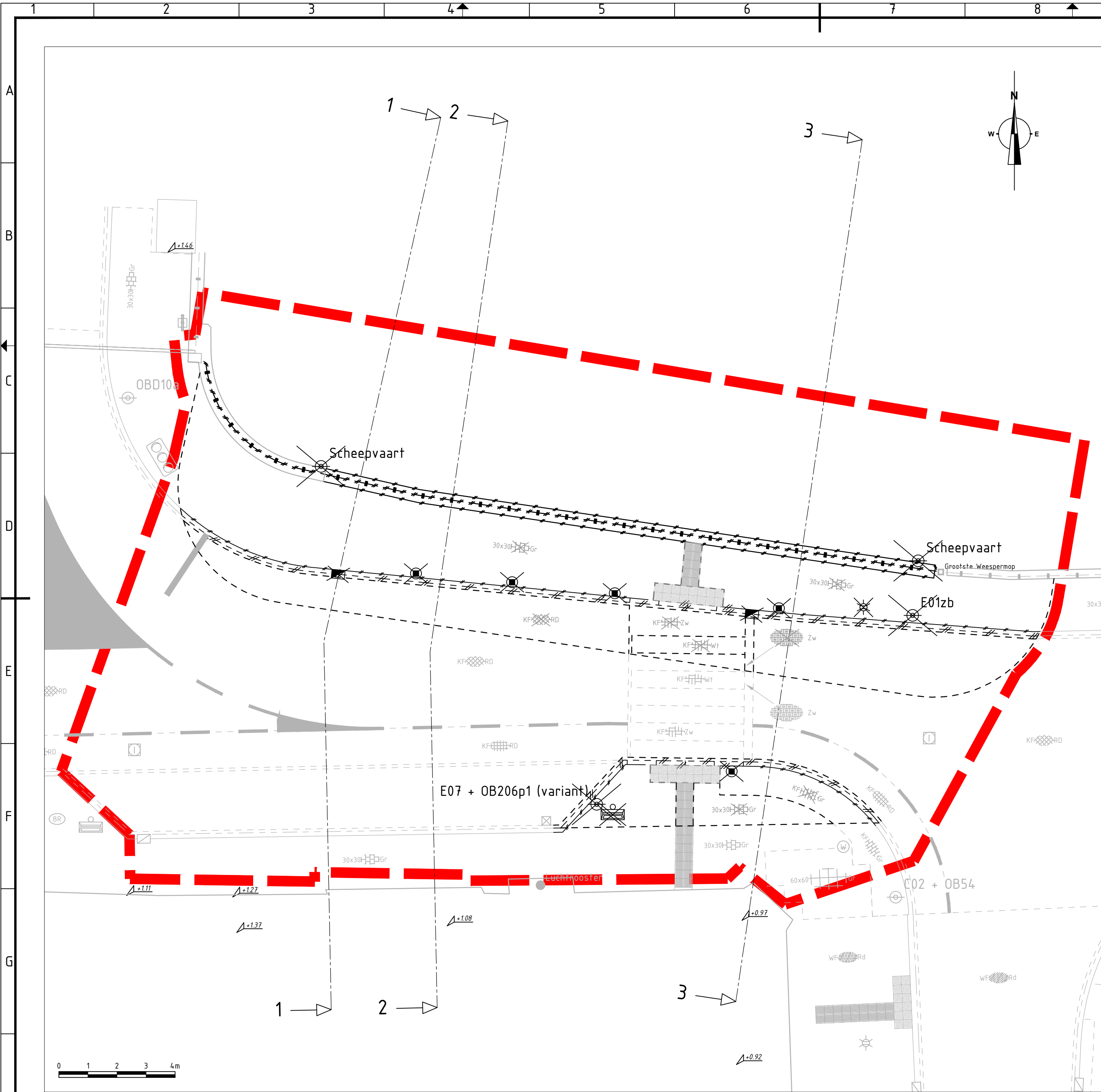
Overzicht op te breken situatie SCHAAL 1 : 100
