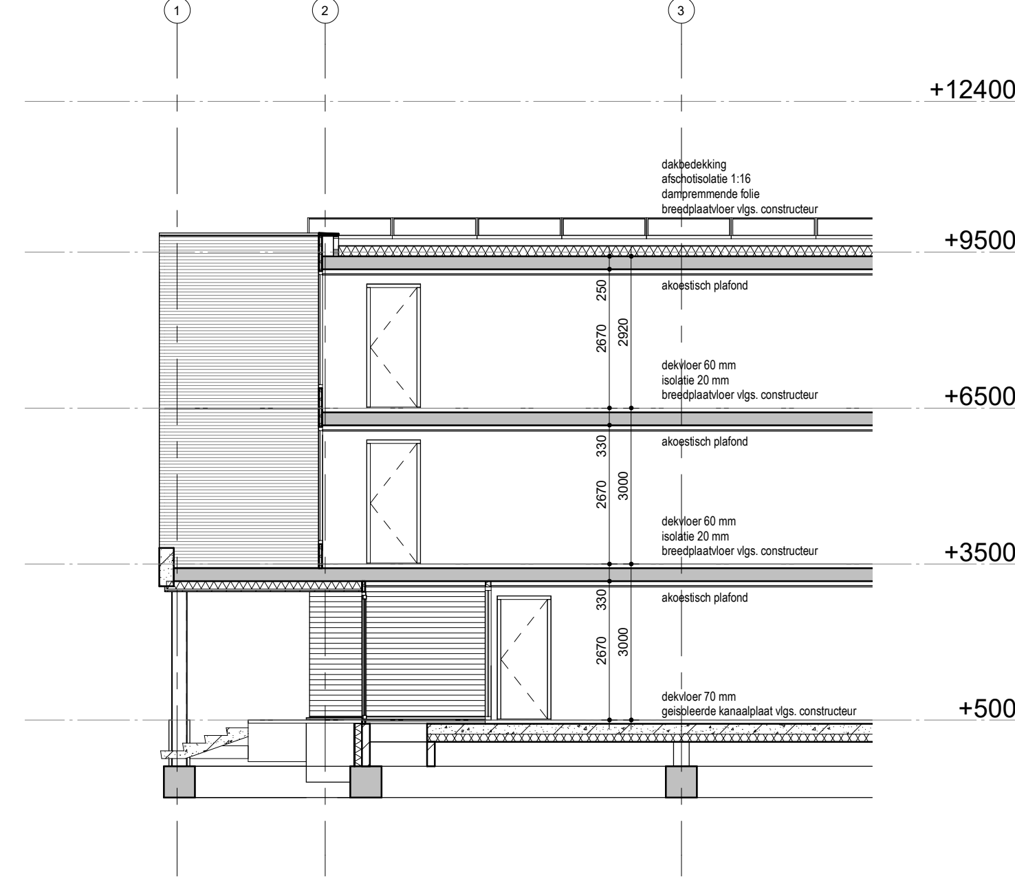
Doorsnede G
