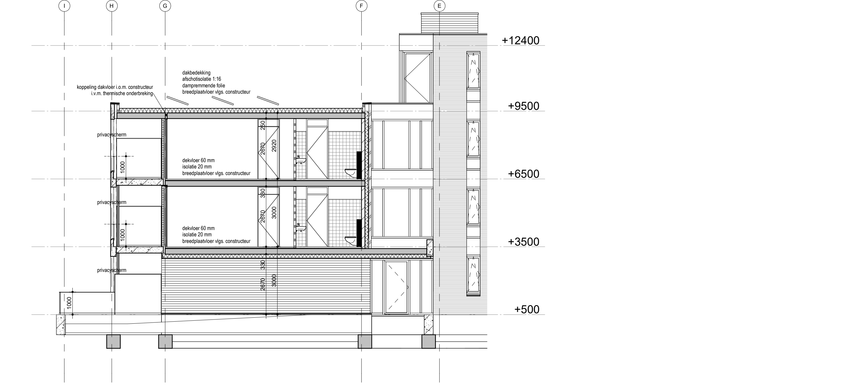
Doorsnede F
