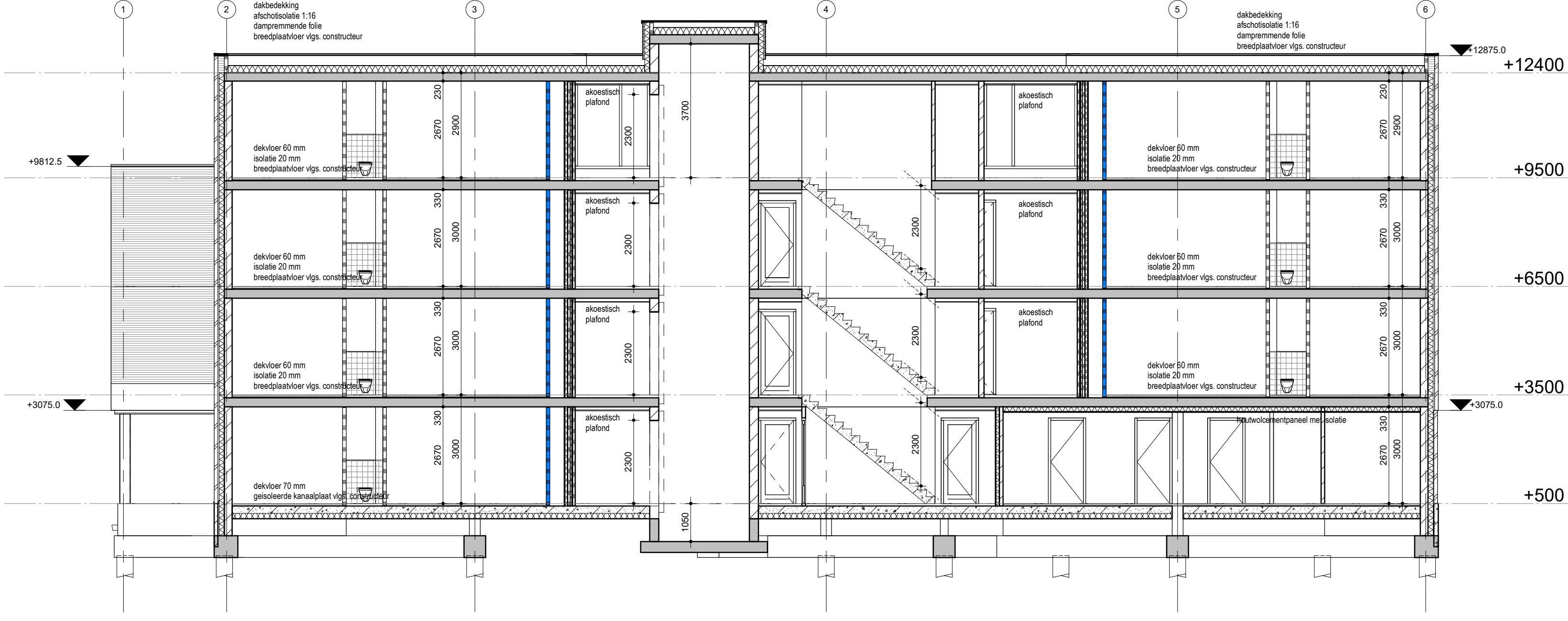
Doorsnede C
