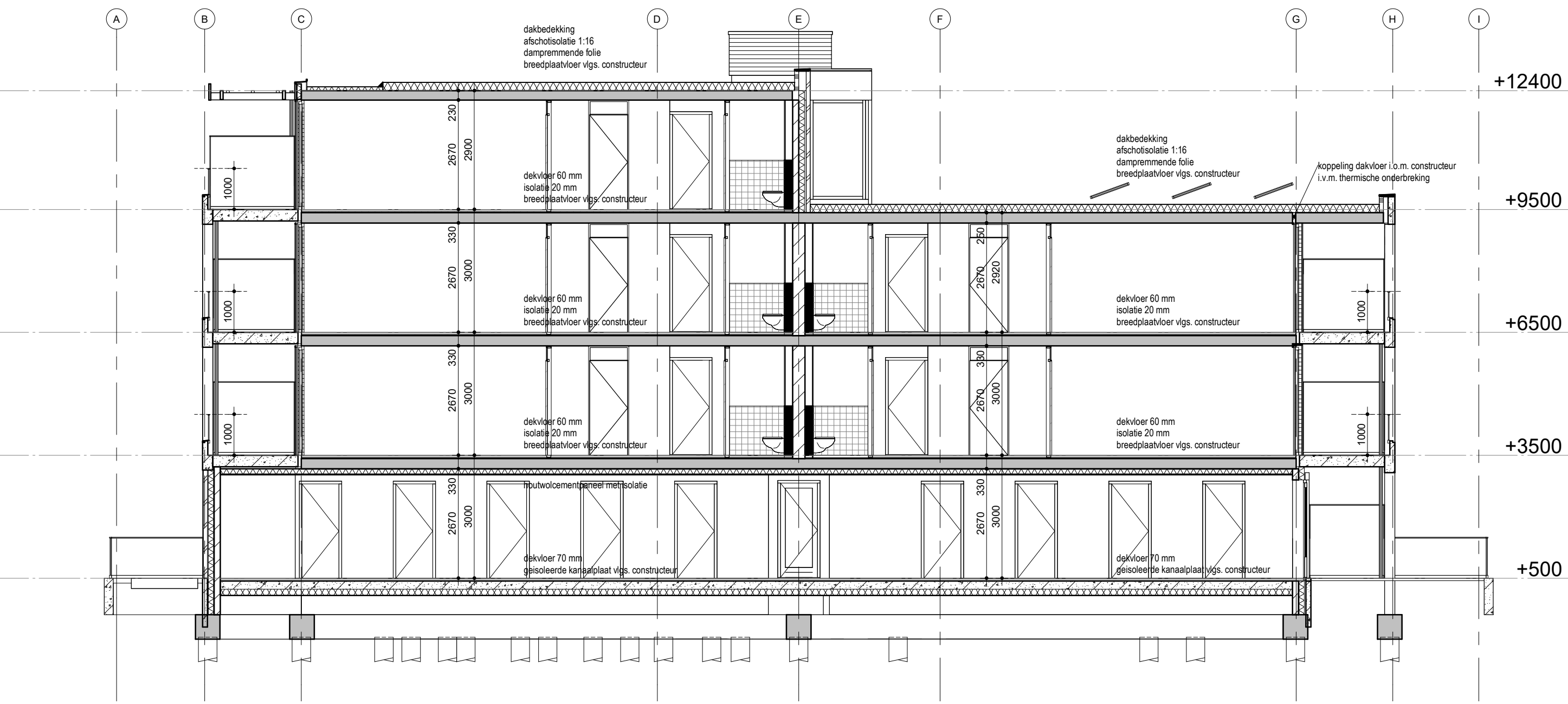
Doorsnede D
