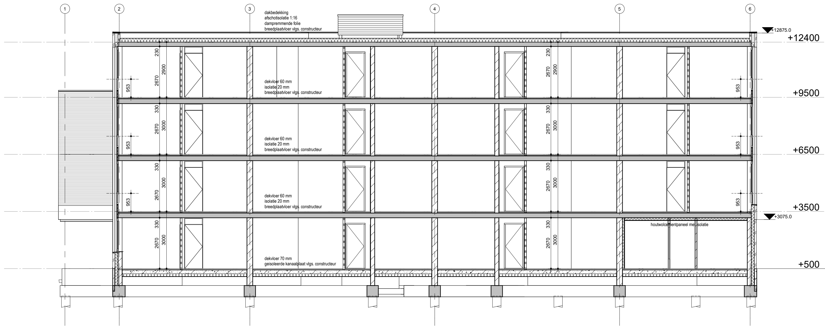
Doorsnede A
