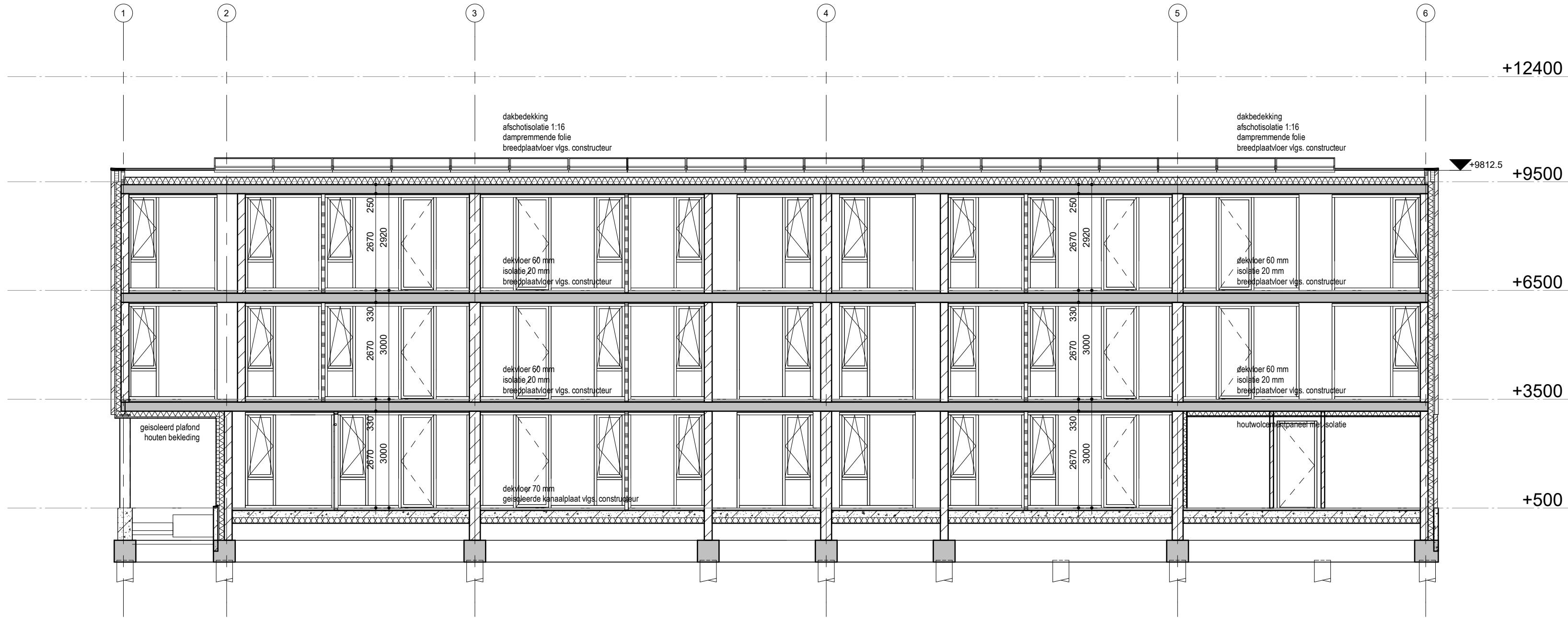
Doorsnede B
