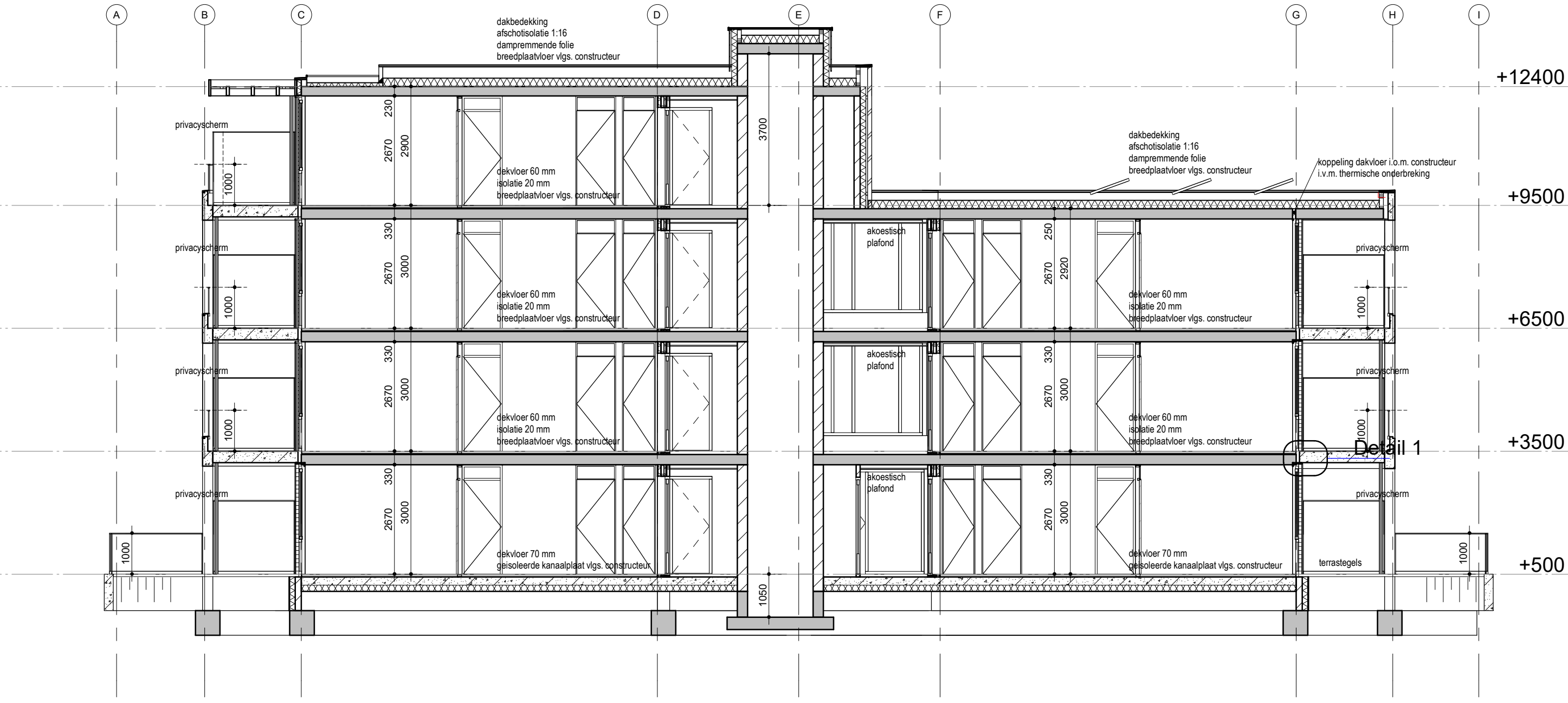
Doorsnede E
