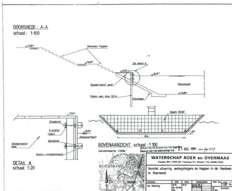
Figuur 1: vergunde steiger
