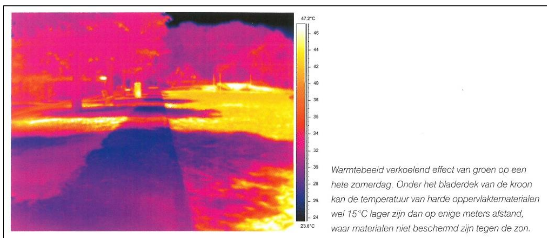
Figuur 4 Warmtebeeld verkoelend effect van groen; rondom de bomen is het koeler (Branchevereniging VHG, 2018)
