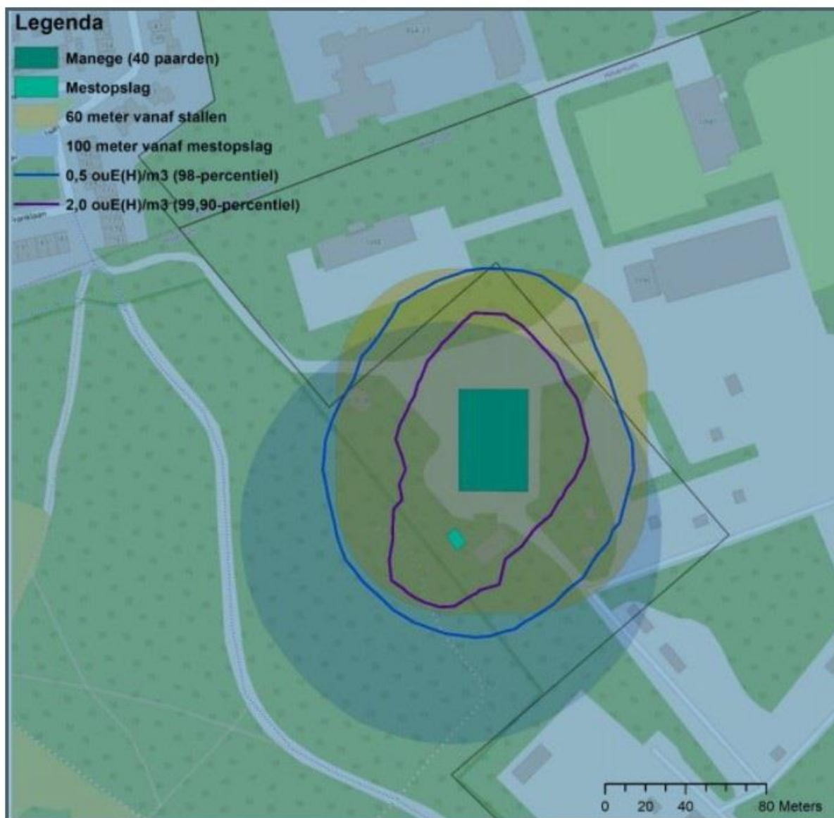
Geurcontouren bij een vaste minimumafstandseis van 60 meter (40 paarden)
