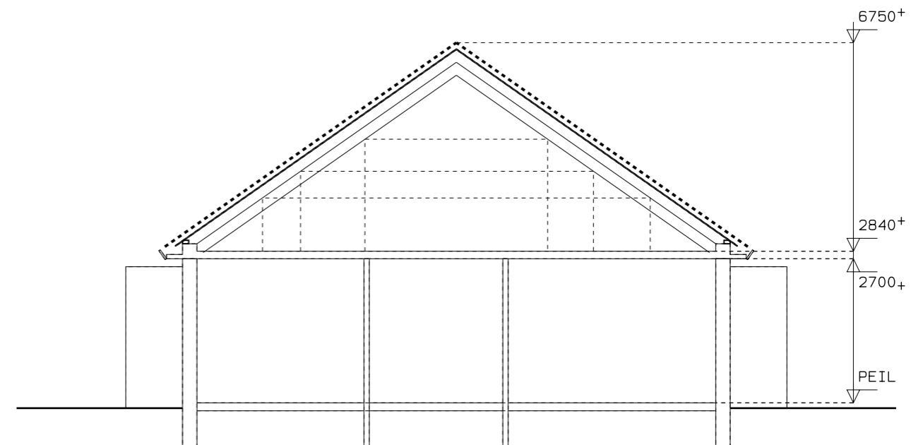
Doorsnede (bestaand)
