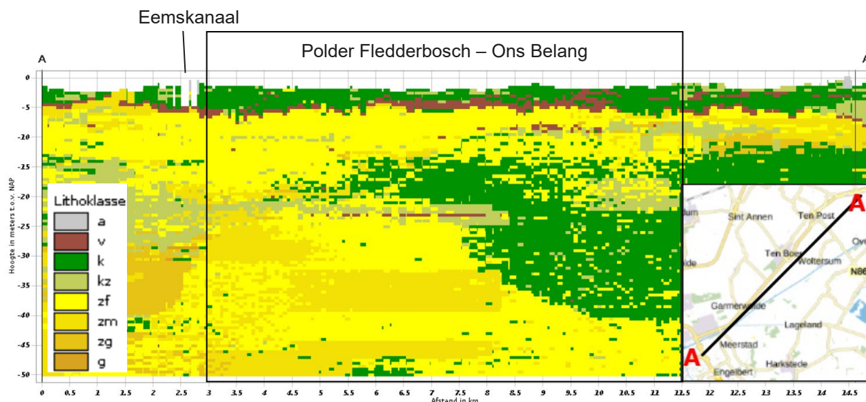
Figuur 8: Verticale doorsnede van de ondergrond uit het model GEOTOP v1.3 (Bron: https://www.dinoloket.nl/ondergrondmodellen ).
