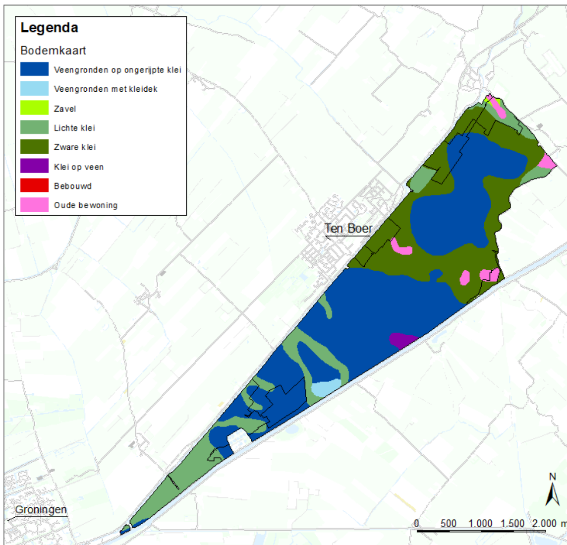
Figuur 7: De opbouw van de bodem (tot circa 1,2 m onder maaiveld). (Bron: De Bodemkaart van Nederland Digitaal, Alterra.)
