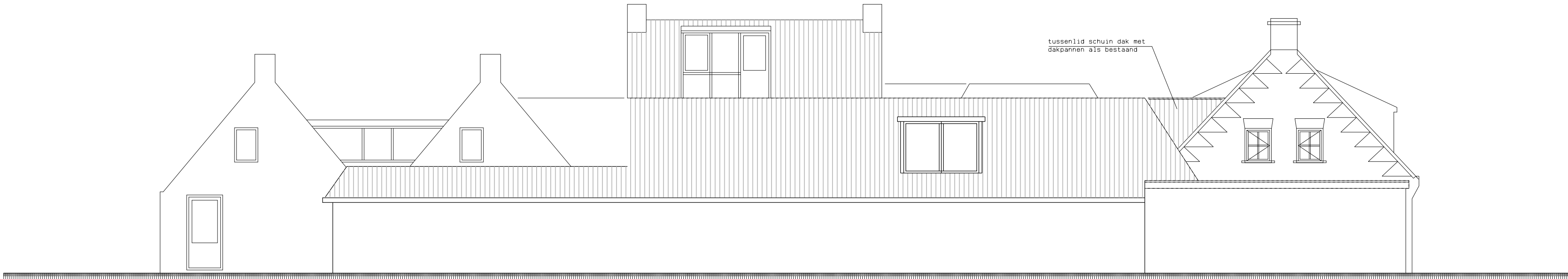
Achtergevel (gewijzigd)
