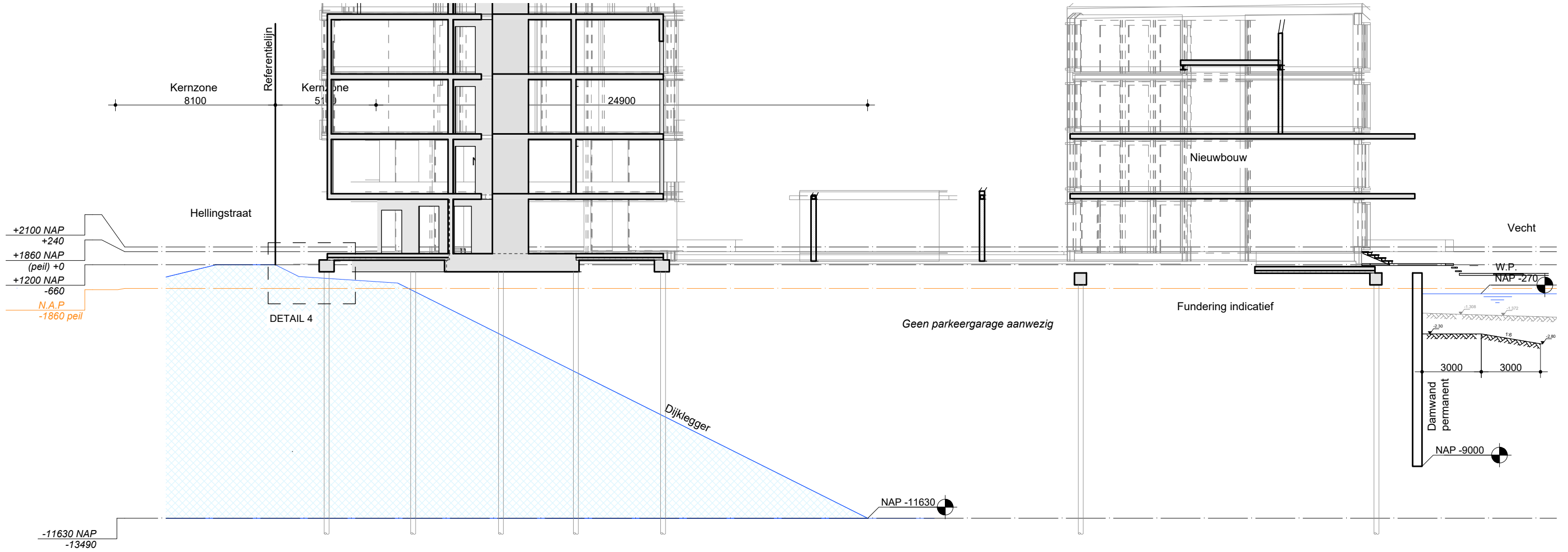
DOORSNEDE 4 1:200
