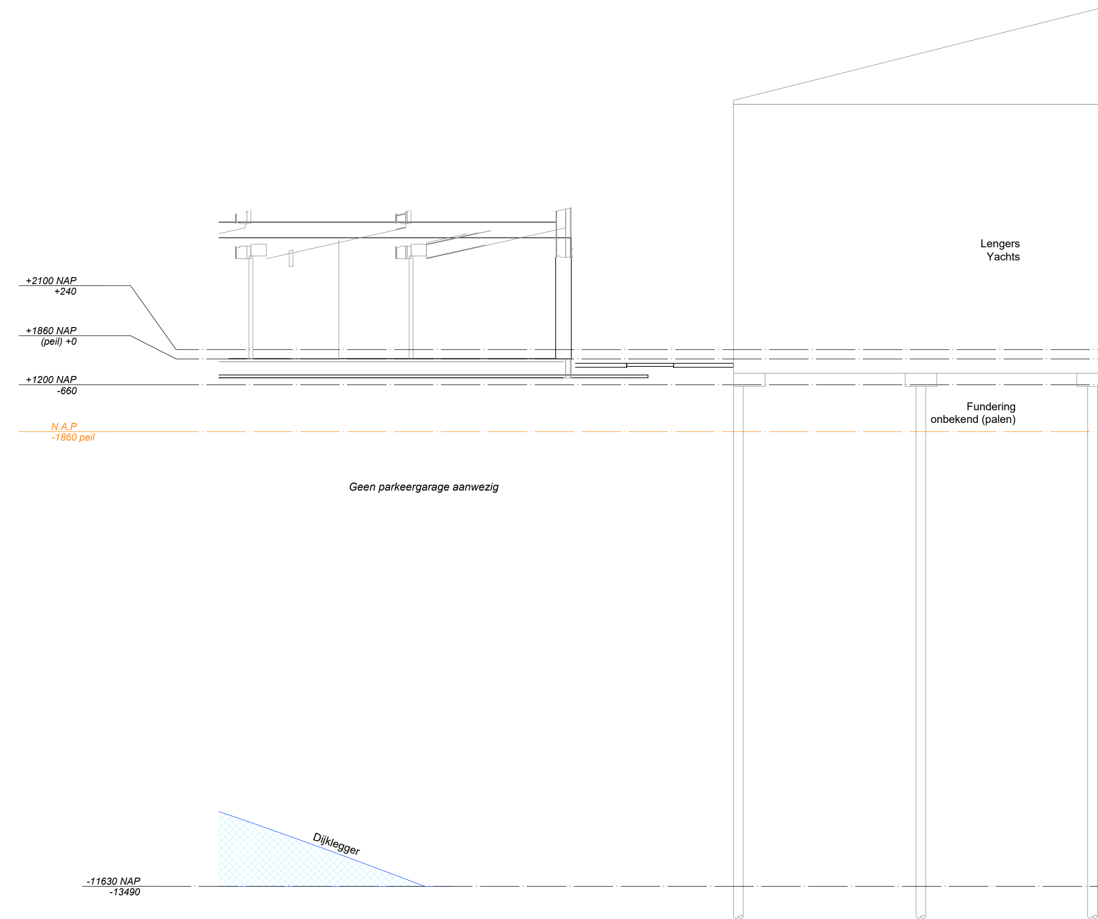
DOORSNEDE 5 1:100
