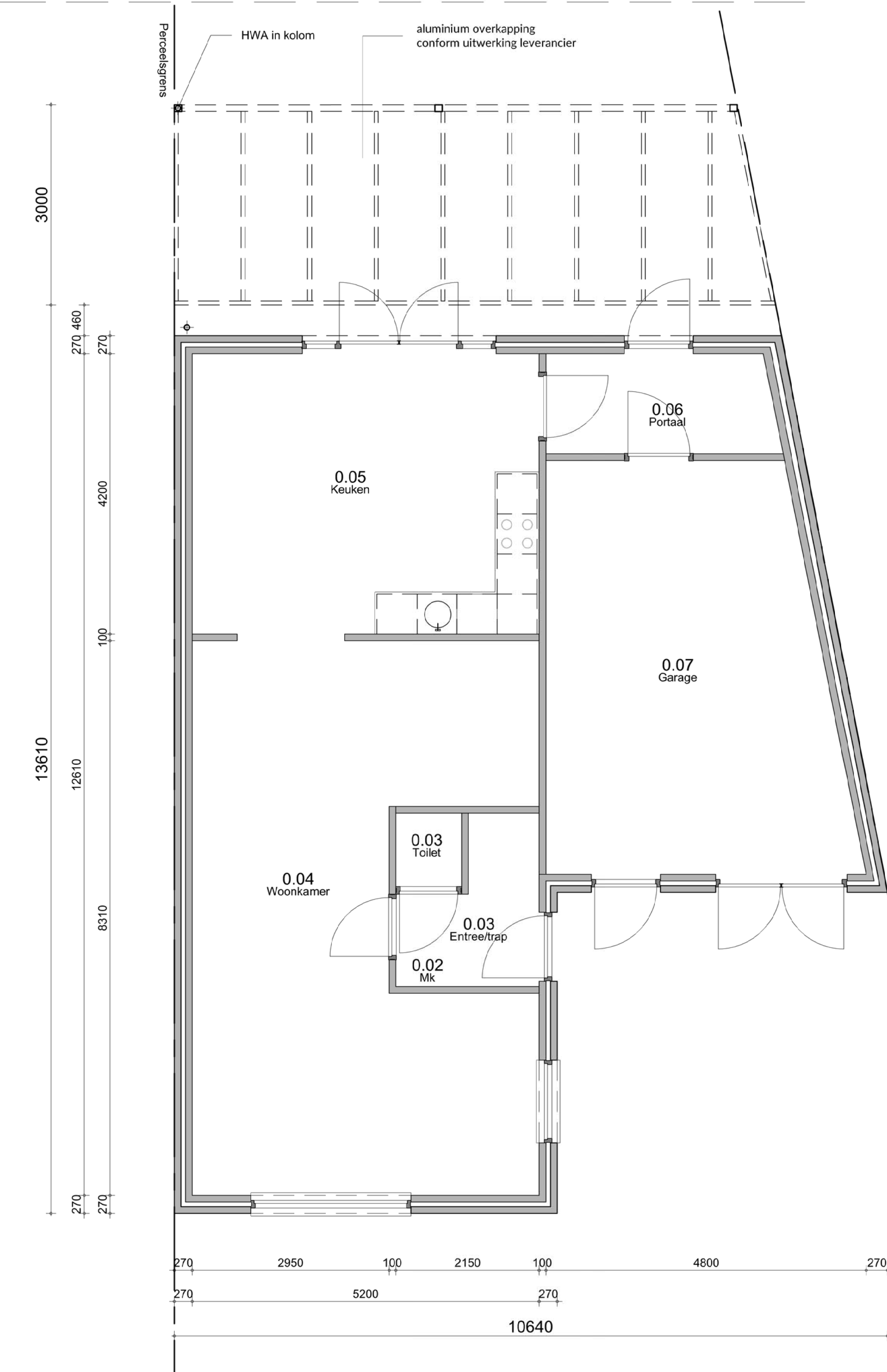
plattegrond begane grond - nieuwe situatie (Peil = 0)
