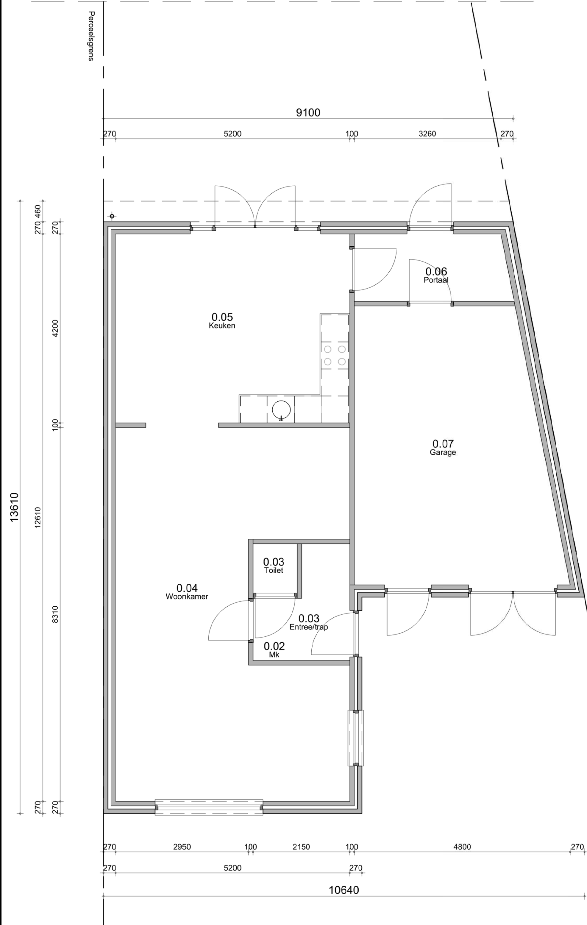
plattegrond begane grond - bestaande situatie (Peil = 0)
