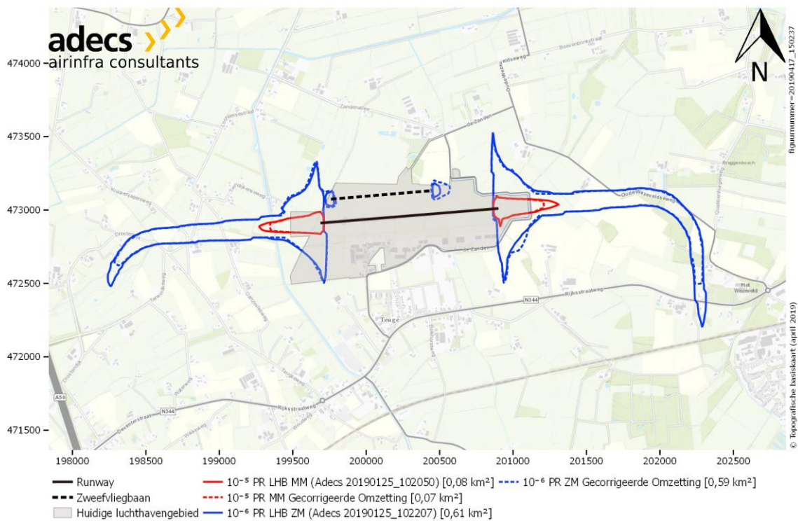
Figuur 5 Ligging 10 -5 en 10 -6 plaatsgebondenrisicocontouren LHB en gecorrigeerde omzetting.
