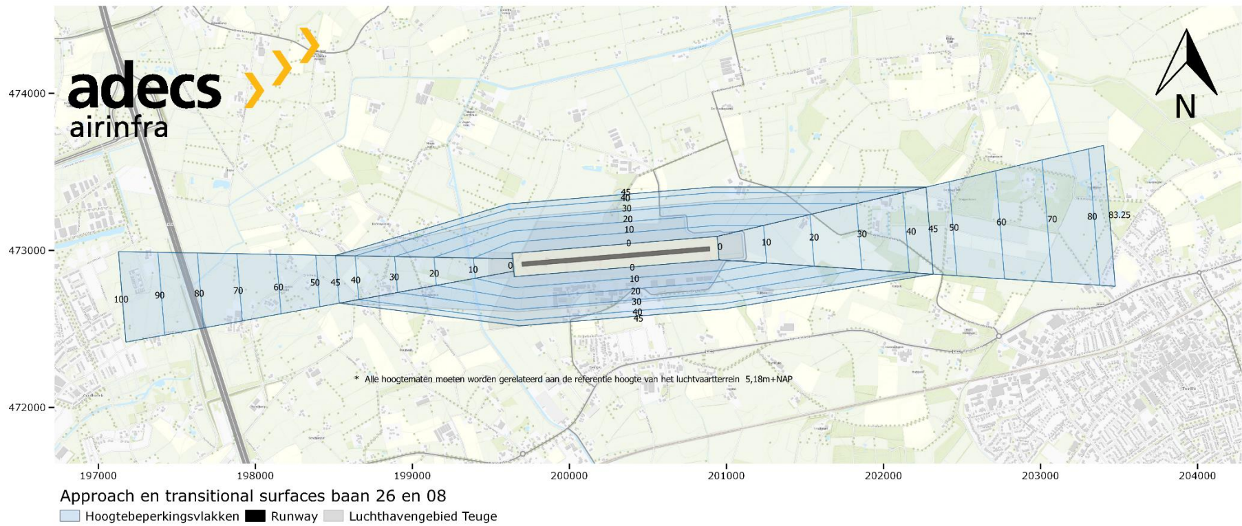
Figuur 11 Approach en transitional surfaces baan 26 en 08.
