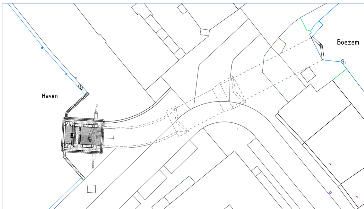
Situatietekening Wateringsesluis
