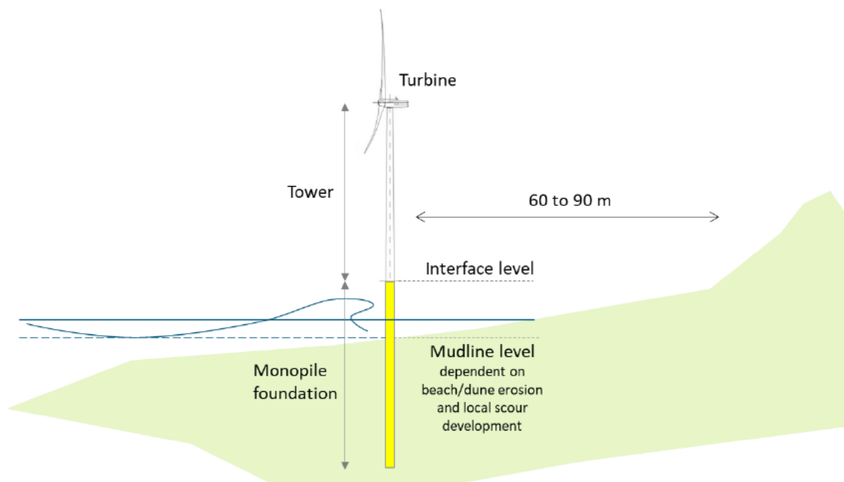
Figuur 2. Conceptueel ontwerp van de monopaal fundering
