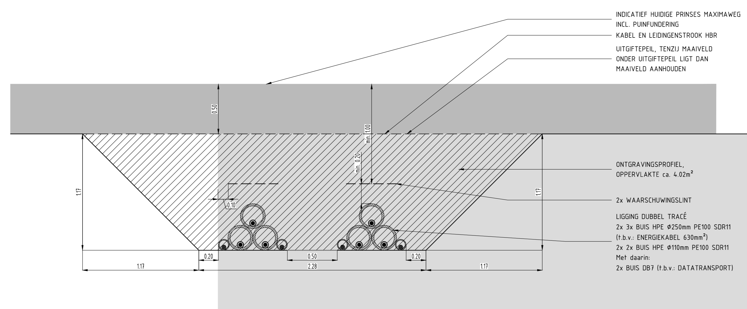
PRINCIPE ONTGRAVINGSPROFIEL 6 DUBBEL LEGTRACÉ KRUISING PRINSES MAXIMAWEG IN HBR STROOK
