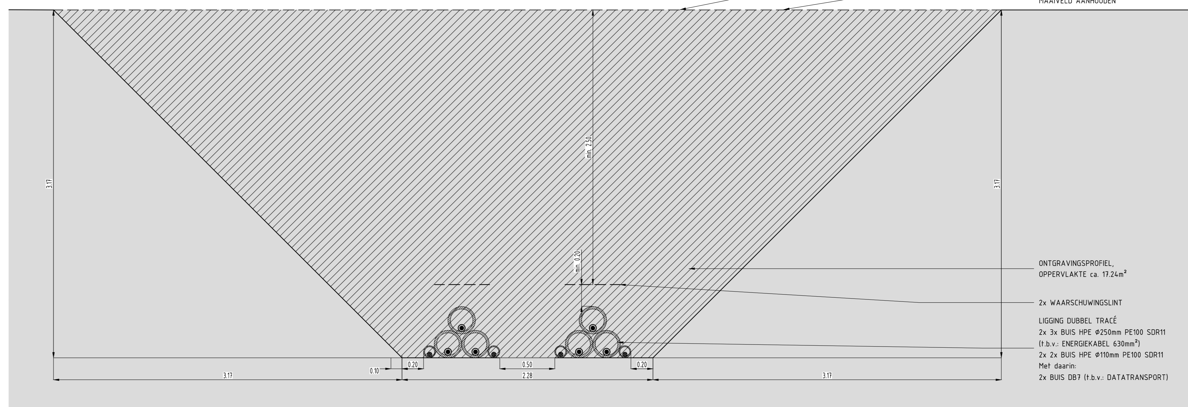
PRINCIPE ONTGRAVINGSPROFIEL 9 DUBBEL LEGTRACÉ KRUISING HBR STROOK
