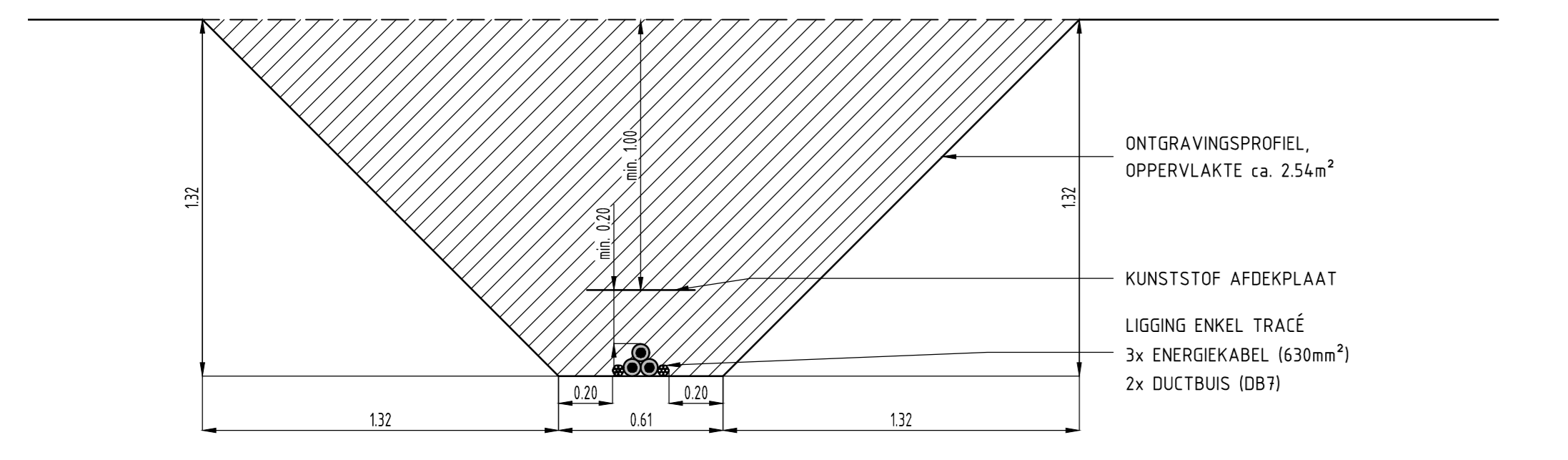
PRINCIPE ONTGRAVINGSPROFIEL 1 ENKEL LEGTRACÉ
