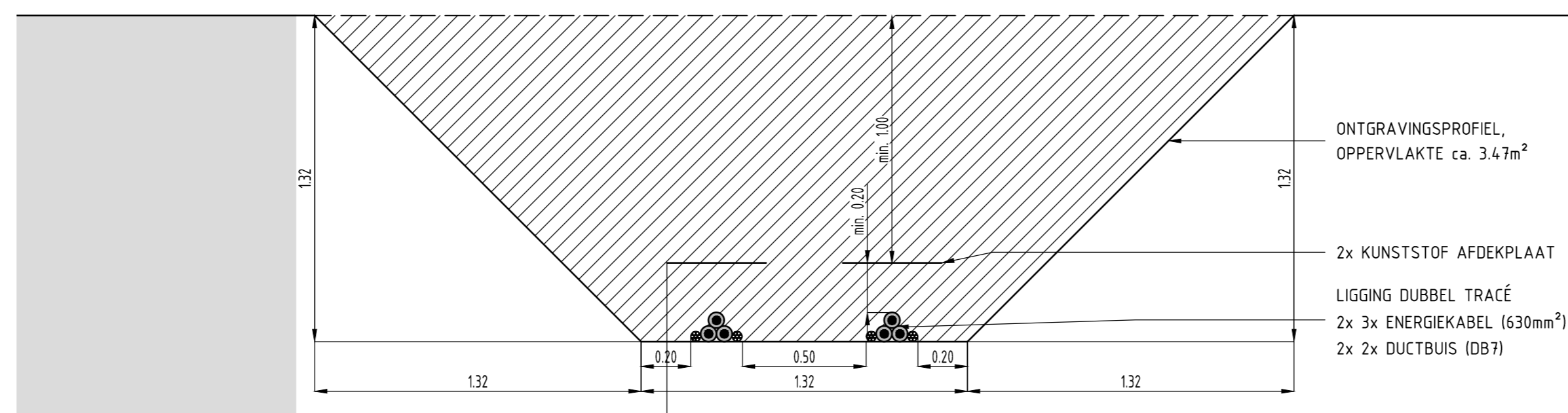
PRINCIPE ONTGRAVINGSPROFIEL 10 DUBBEL LEGTRACÉ PARALLEL AAN HBR STROOK
