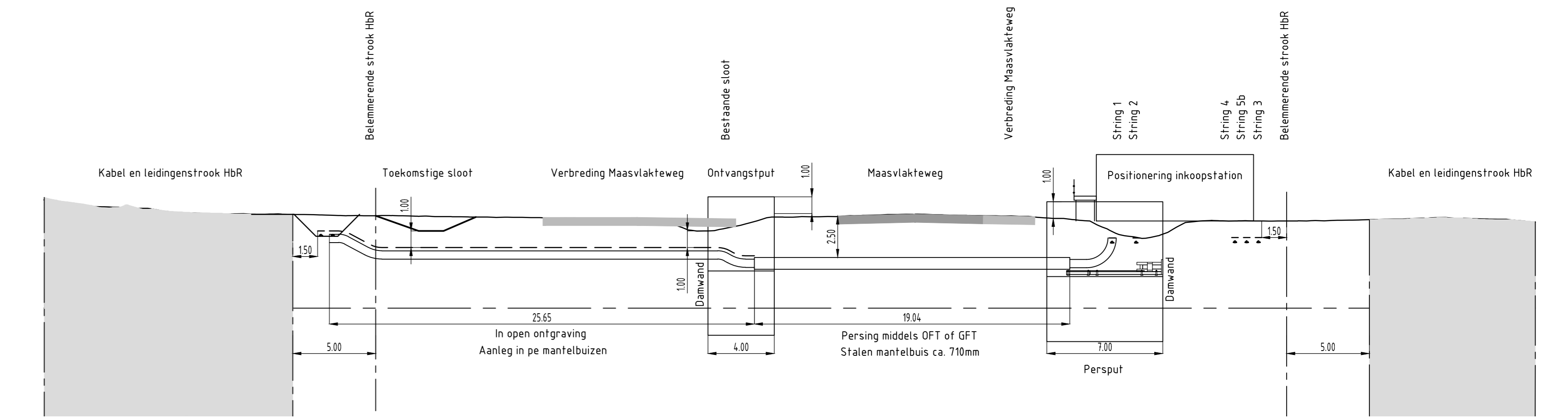
DOORSNEDE A-A PRINCIPE PROFIEL KRUISING MAASVLAKTEWEG MIDDELS GFT/OFT EN OPEN ONTGRAVING
