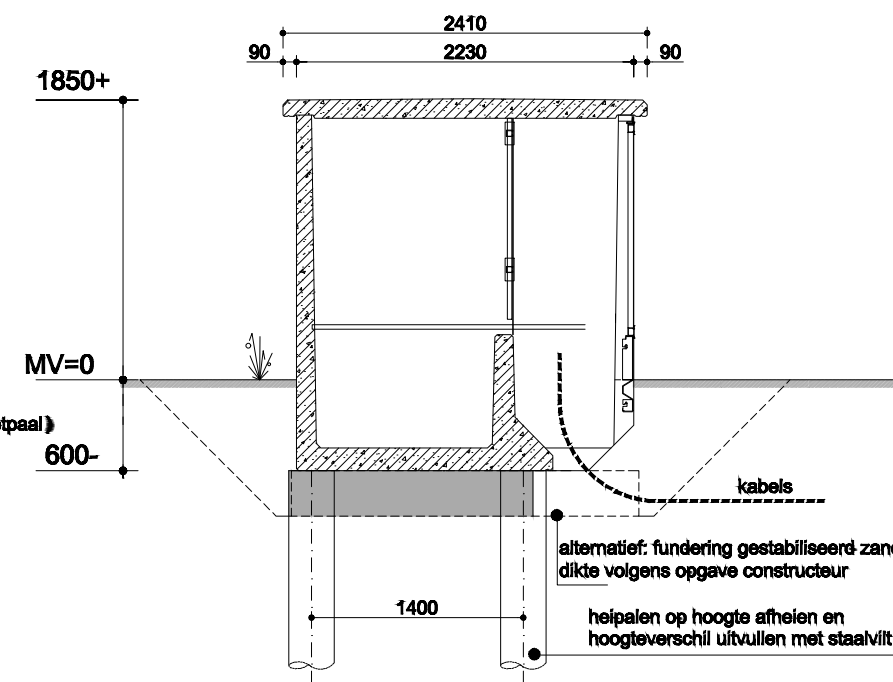
DOORSNEDE D-D
