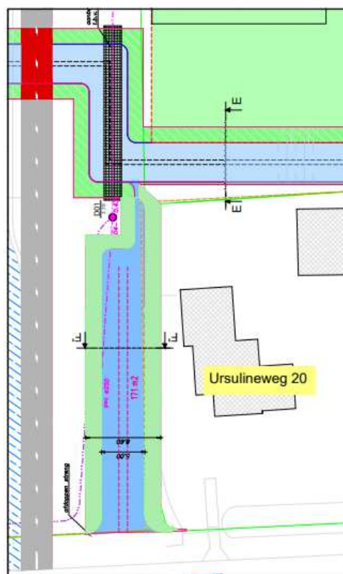
Bovenaanzicht van de te vergroten watergang
