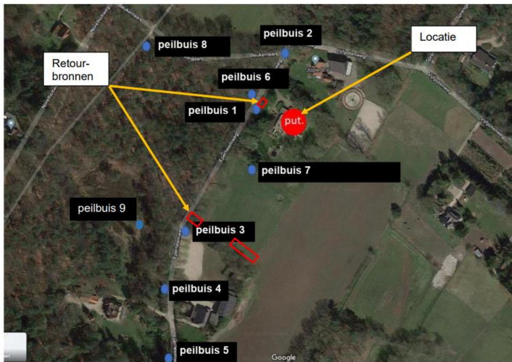
Monitoringspeilbuizen
