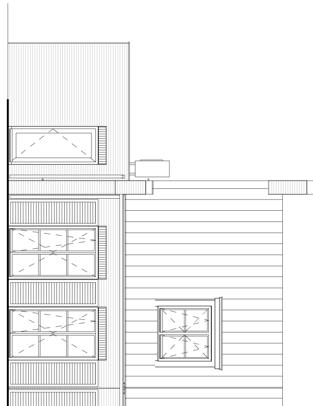
OPTIE DAKKAPEL 1500
