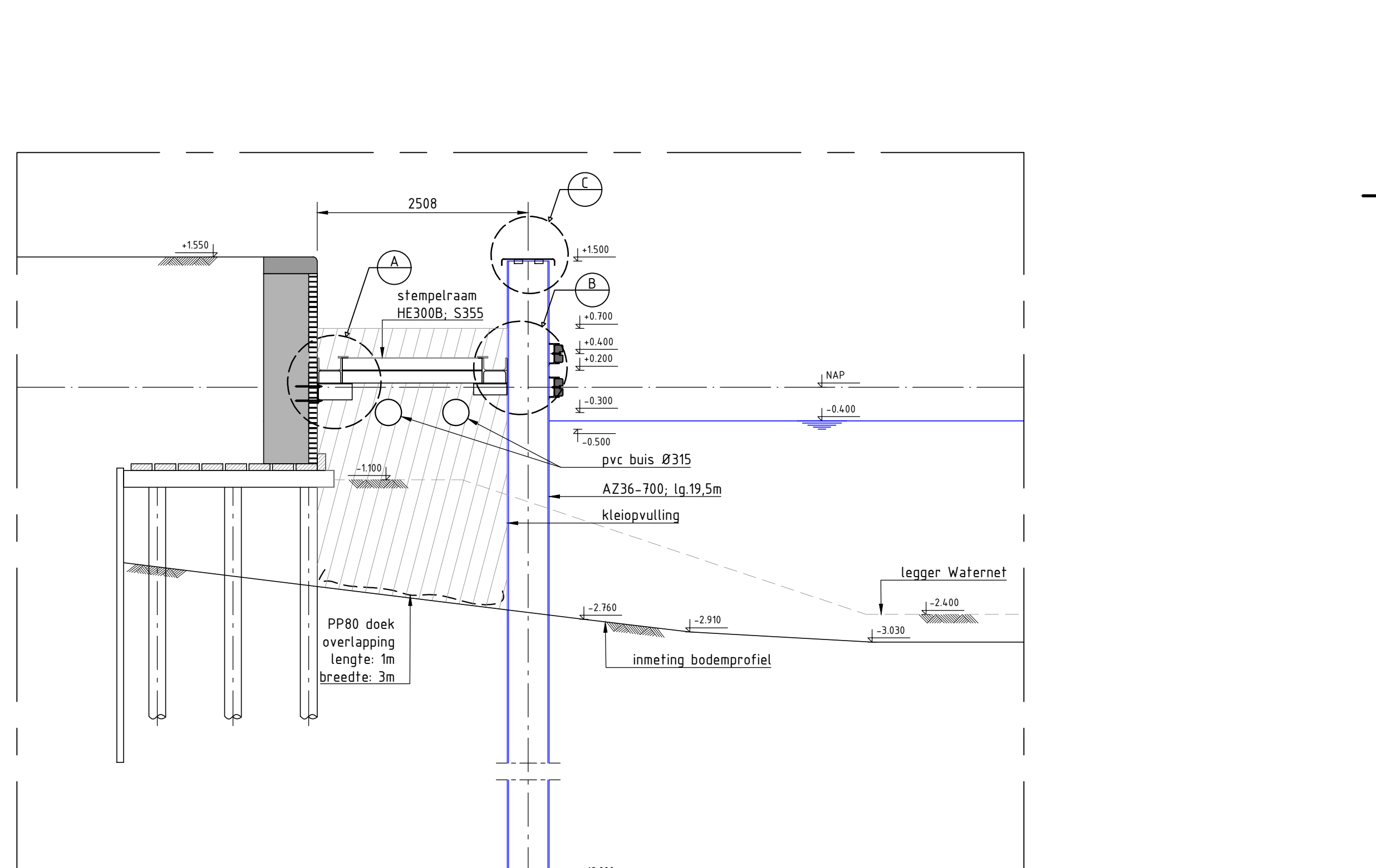
DOORSNEDEN B-B SCHAAL 1: 50
