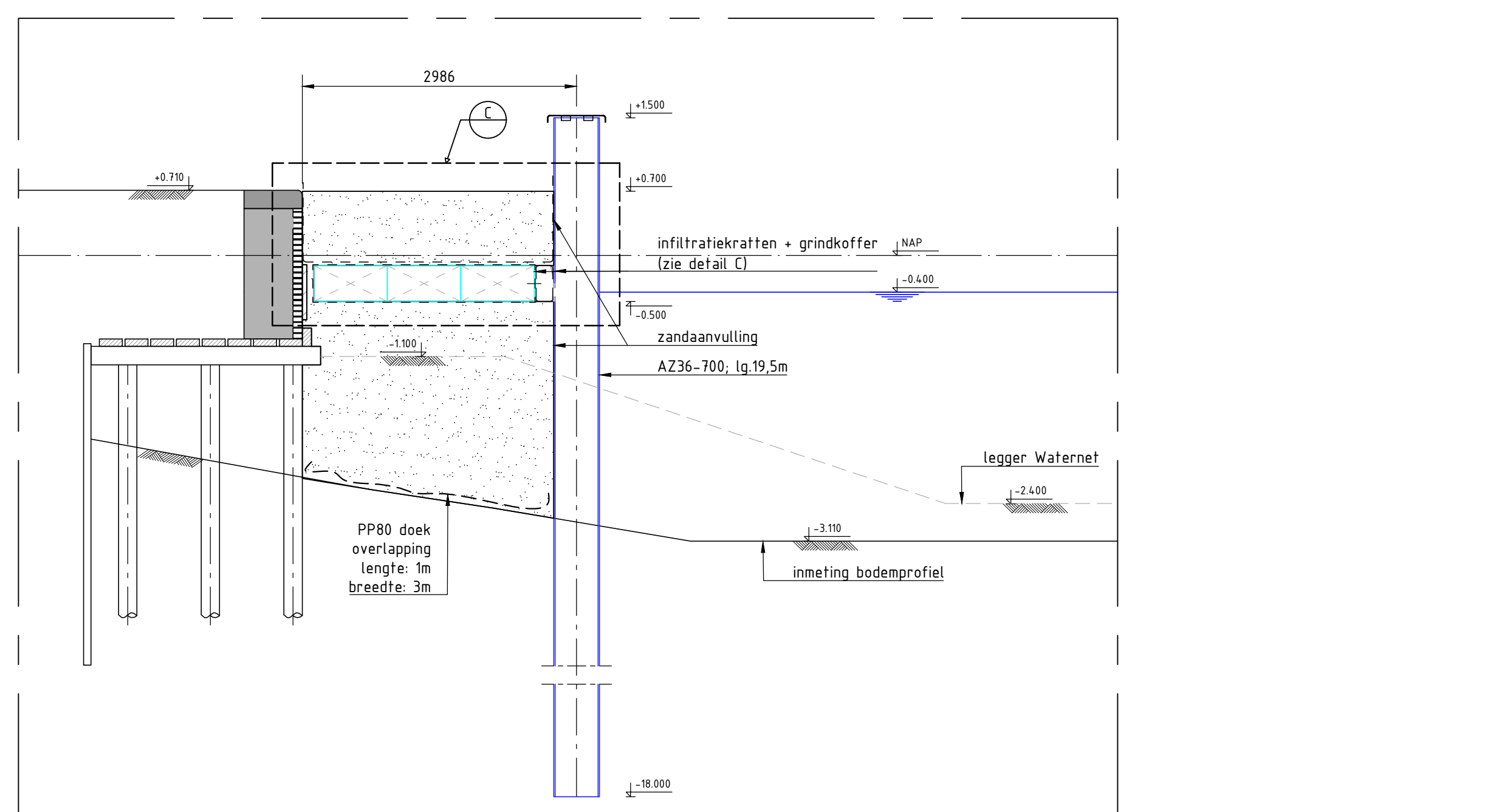
DOORSNEDEN A-A SCHAAL 1: 50
