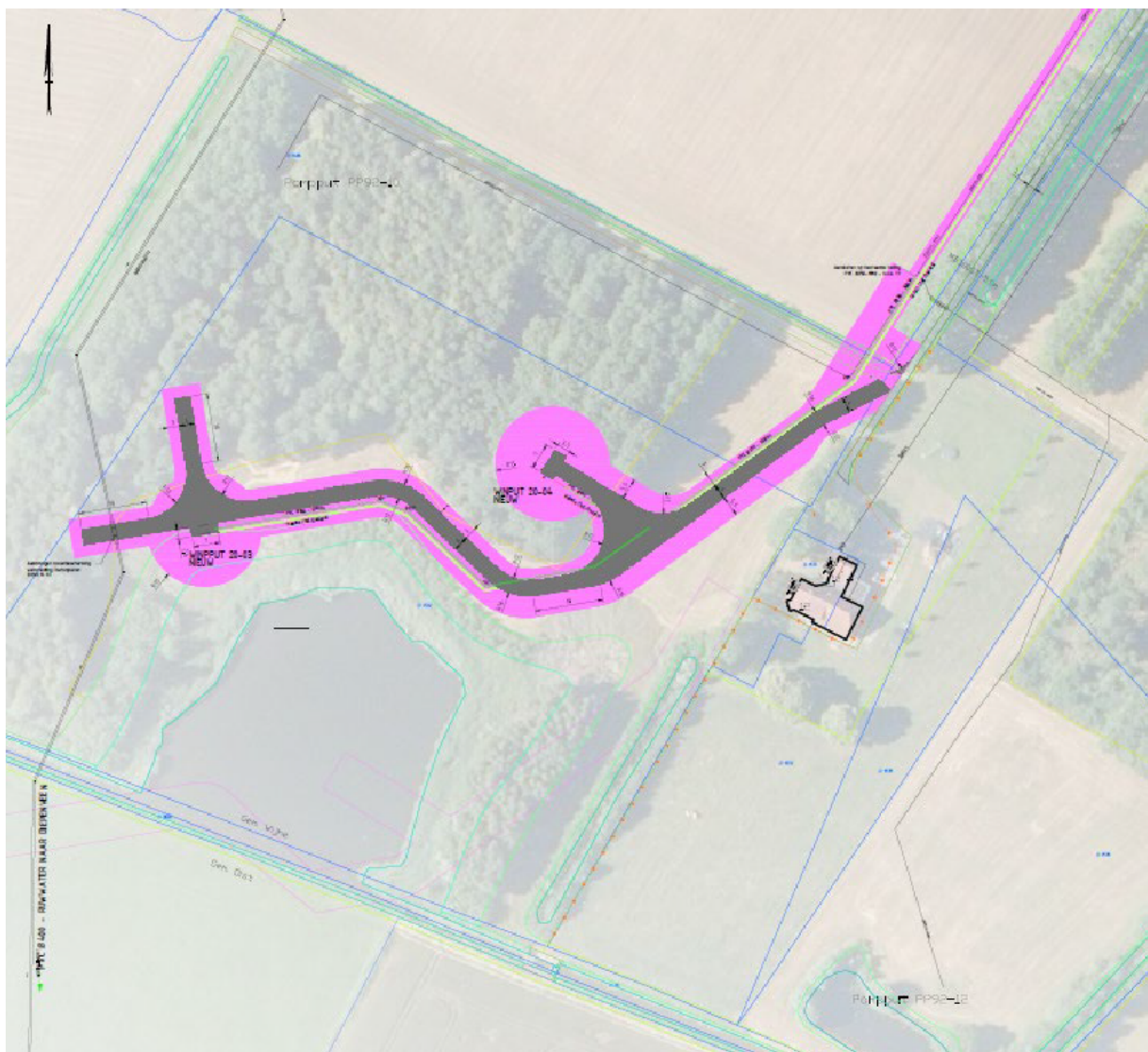
Figuur 2. Geplande werkzaamheden binnen het zuidelijke gedeelte van het plangebied te Boerhaar. Hierbij worden verhardingen aangelegd waarvoor een werkvlak noodzakelijk is (roze). Binnen dit werkvlak kunnen de geplande werkzaamheden worden uitgevoerd zoals het aanleggen van deze verhardingen en het boren van winpunten (cirkels). Voor het creëren van deze benodigde ruimte binnen het werkvlak moeten ook enkele bomen worden gekapt.
