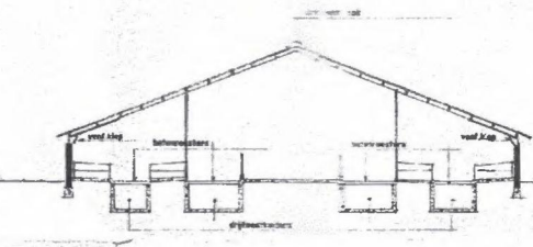
doorsnede geb. 2 a-a
