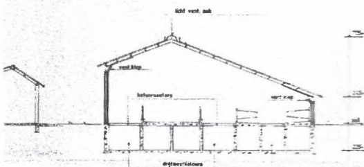
doorsnede geb. 2 b-b
