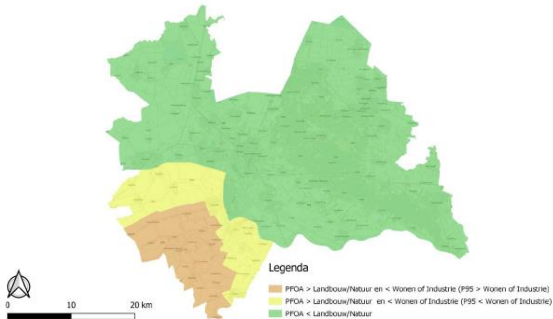
Figuur 2: PFOA bovengrond (0,0 – 0,5 m-mv)
