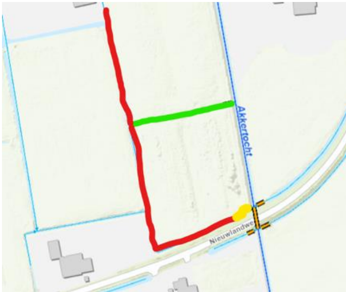
Figuur 1: locatie van de werkzaamheden met in het rood aangegeven de te verbreden watergang, in het groen de te dempen watergang en in het geel de te verlengen dam met duiker.
