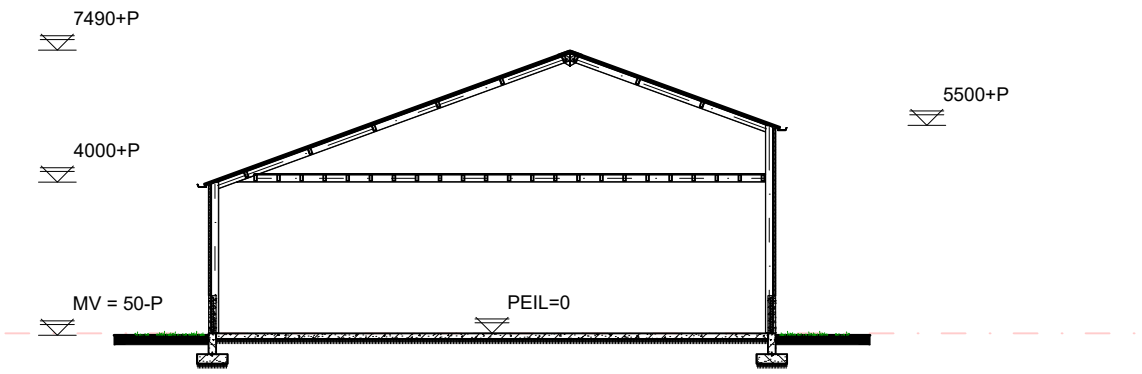
DOORSNEDE A-A GEBOUWNR 1
