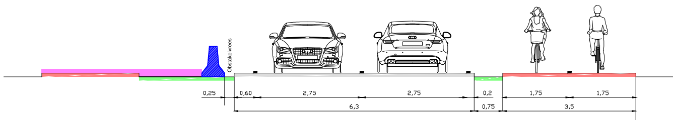
Dwarsprofiel A Schaal: 1:100
