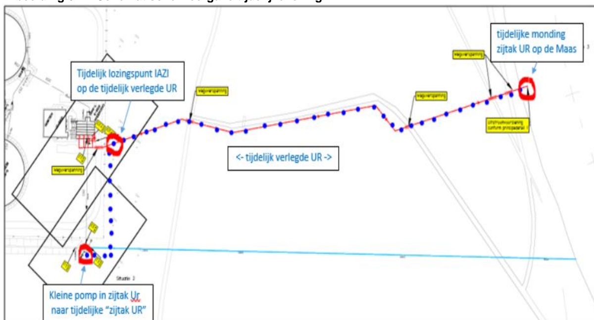
Afbeelding 6-1 Schematische weergave tijdelijke lozing
