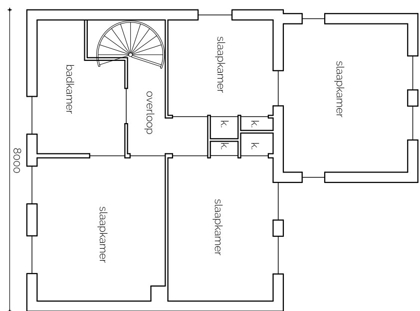
bestaande verdieping
