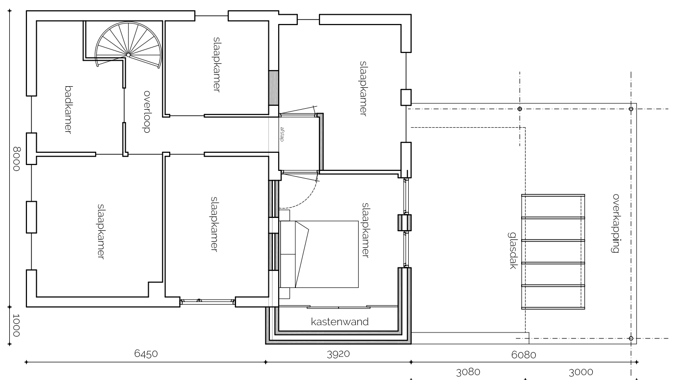
nieuwe verdieping
