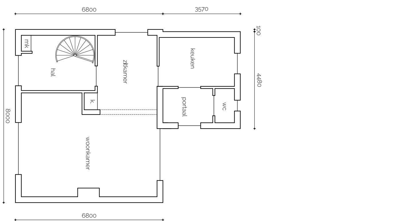
bestaande beganegrond
