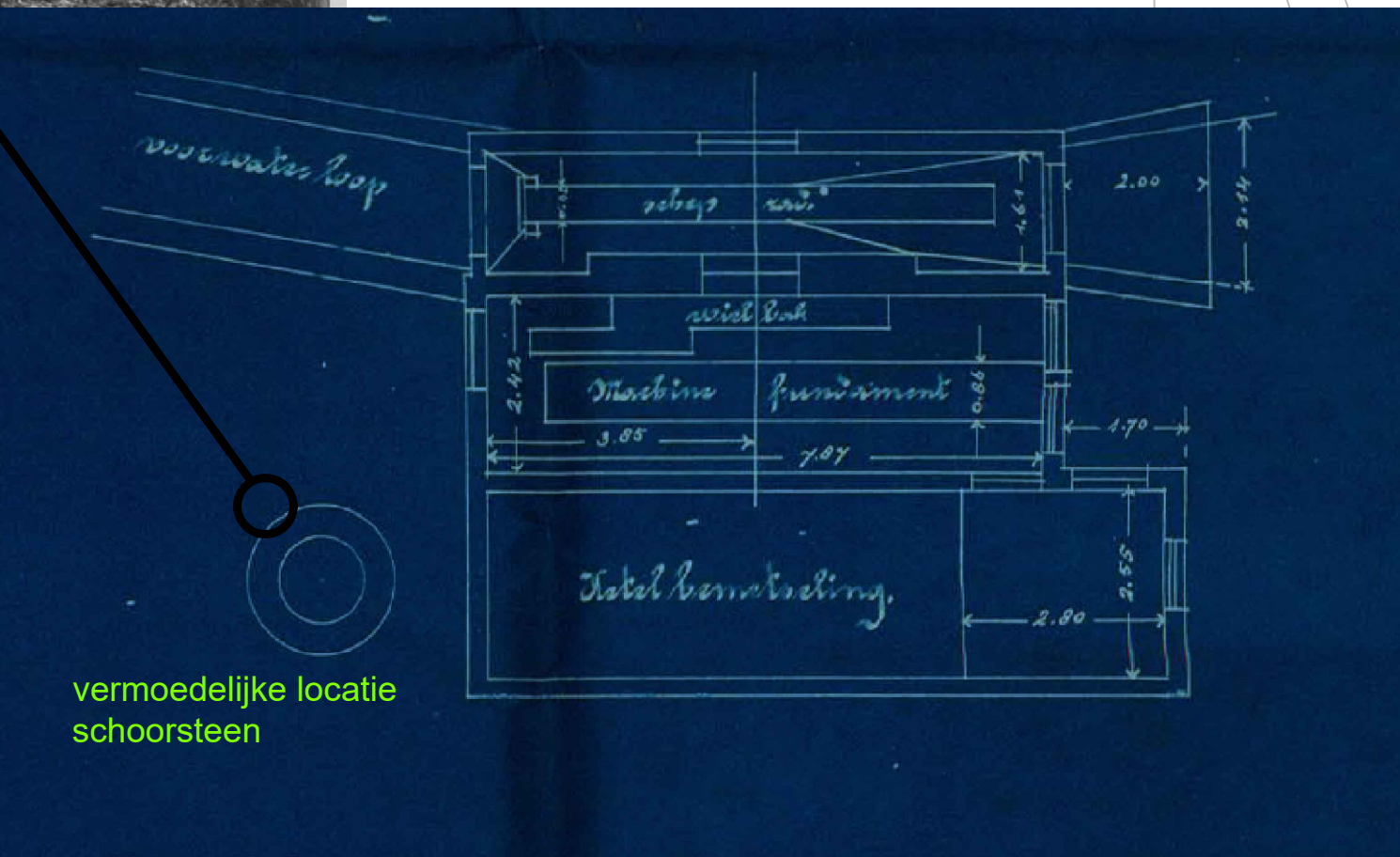
tekening ombouw naar elektrisch gemaal 1919 (let op; gemaal gespiegeld)
