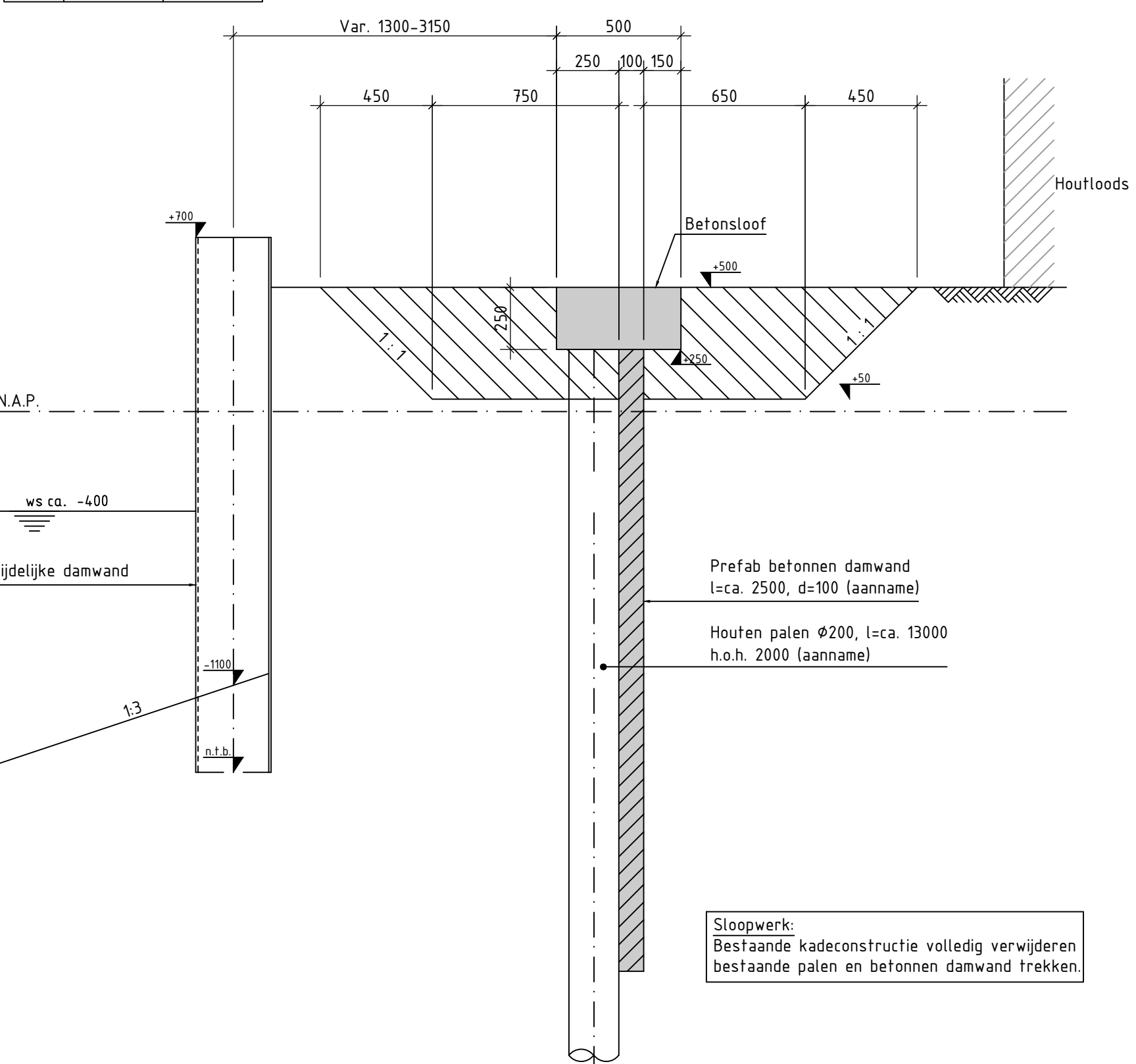
DOORSNEDEN A SCHAAL 1 : 20 BESTAAND
