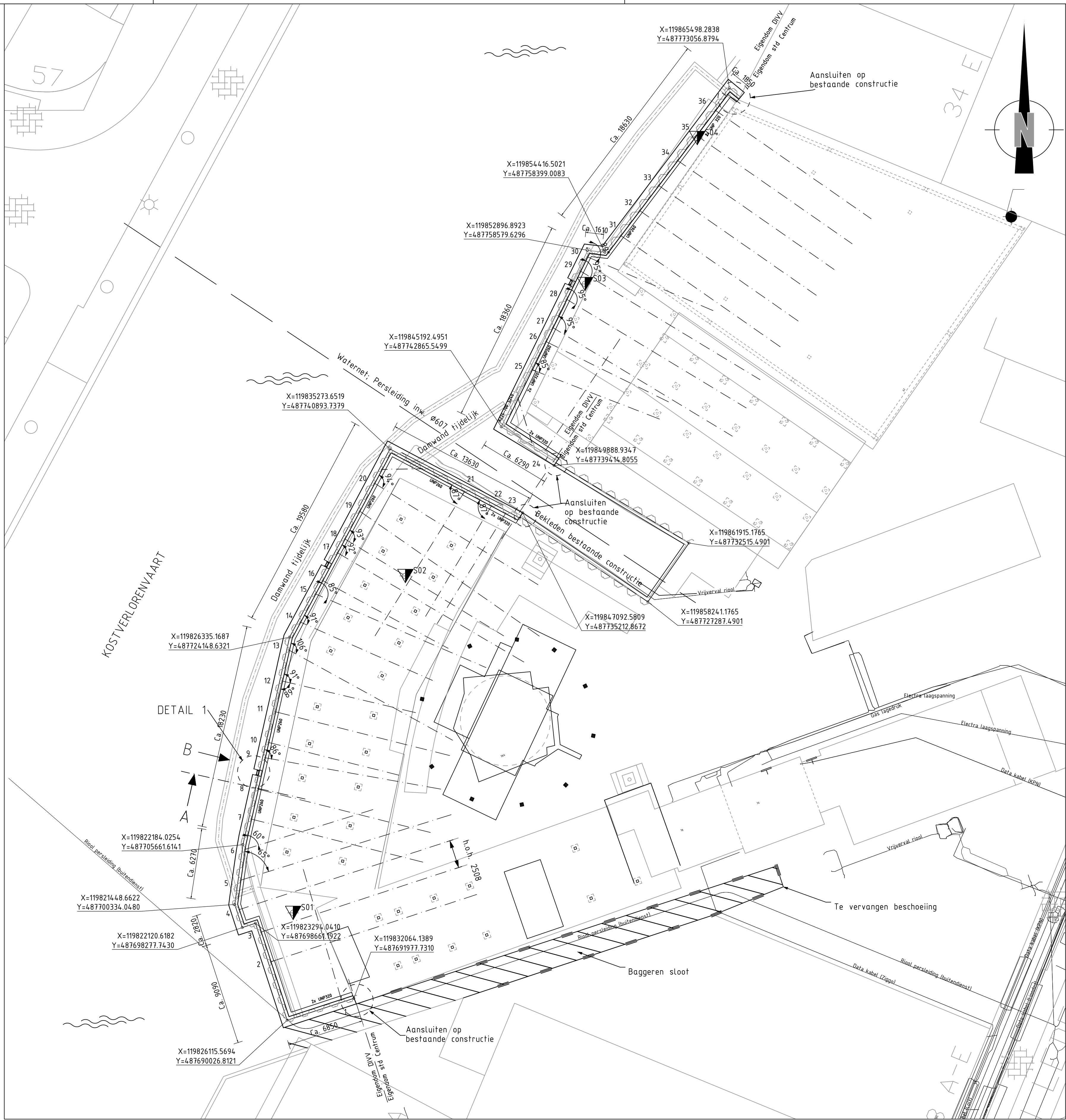
BOVENAANZICHT NIEUW SCHAAL 1 : 200
