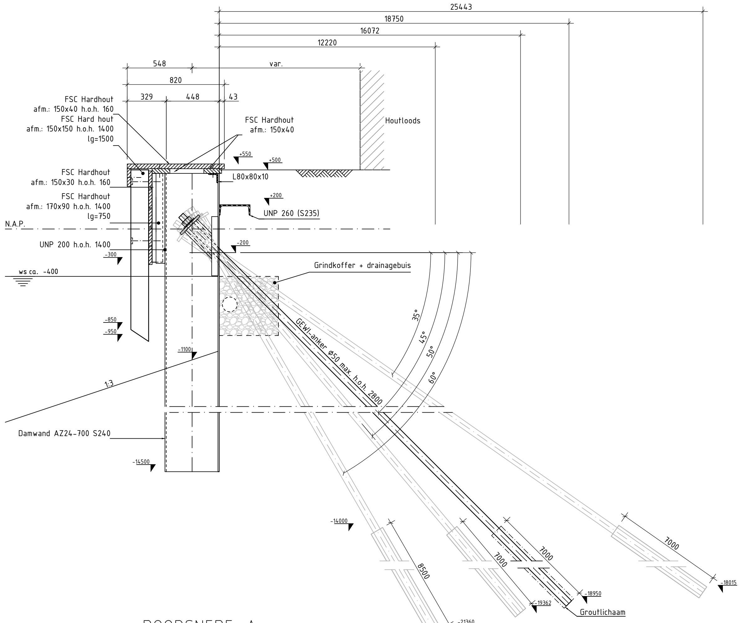
DOORSNEDEN A SCHAAL 1 : 20 NIEUW
