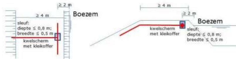
Figuur 2.1 Middels een open sleuf aanleggen van kabels, leidingen ( \leq 63 mm) of mantelbuizen / drukloze leidingen ( \leq 160 mm)
