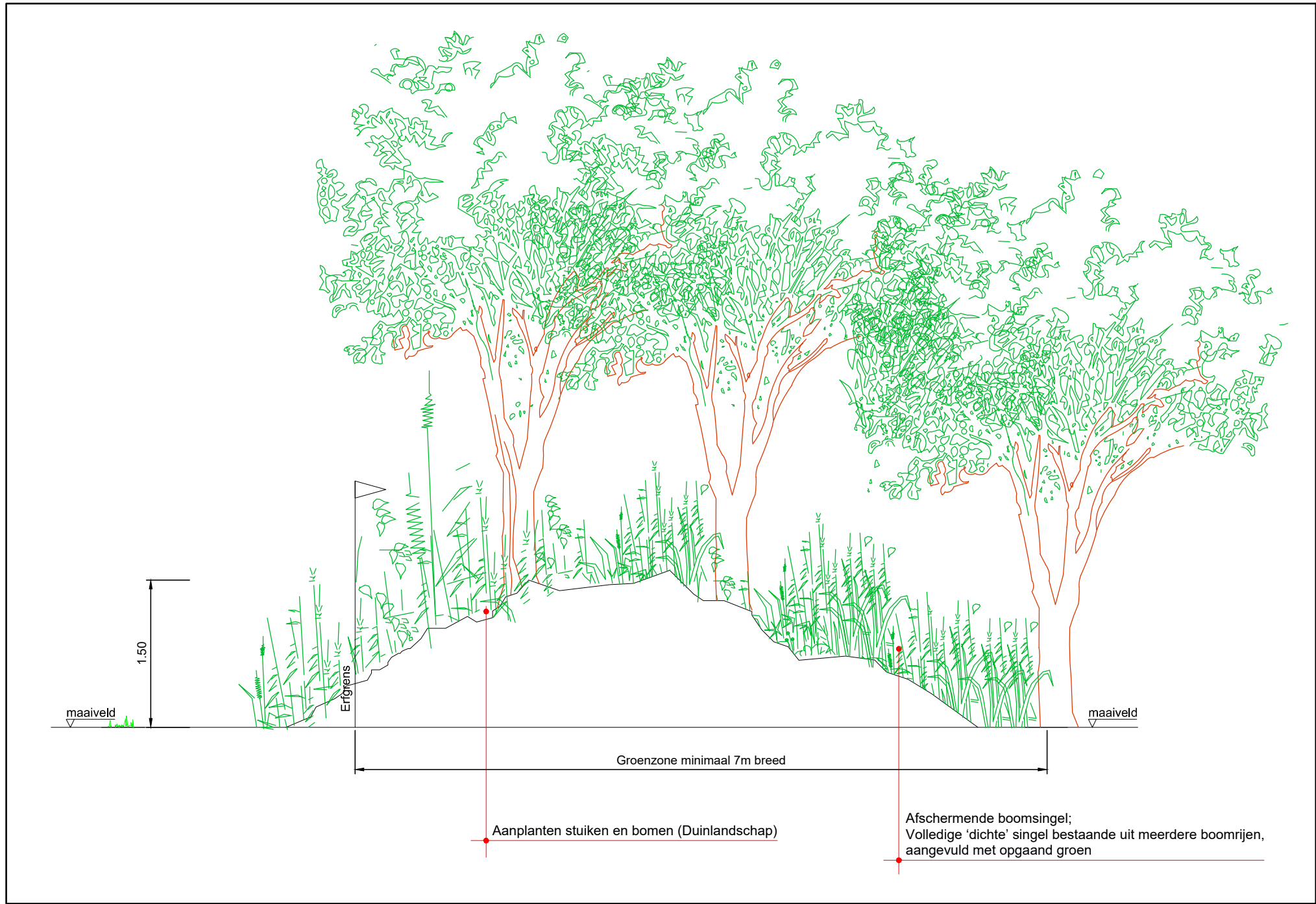
Principe Detail 01 - Ontwerp Wal met Duinlandschap Schaal 1:50
