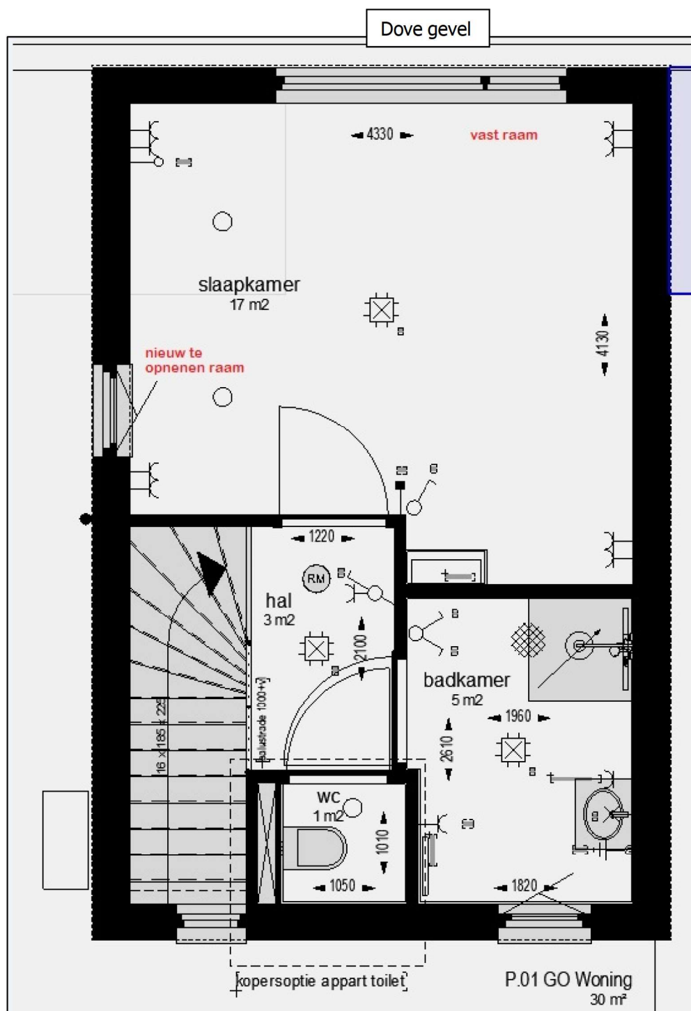
Figuur 2: Creatie dove gevel 1 e verdieping patiowoning
