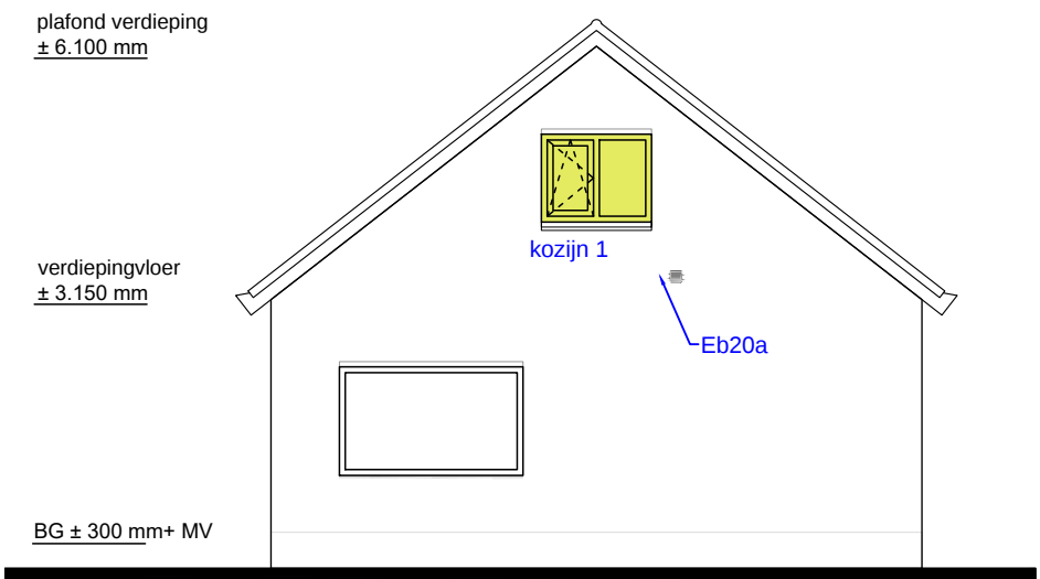
Zijgevel (noord-west zijde) gewijzigde toestand
