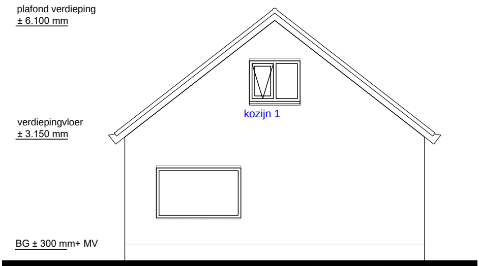
Zijgevel (noord-west zijde) huidige toestand
